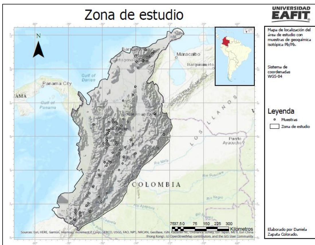
Figura 1. Localización datos de geoquímica isotópica Pb/Pb utilizados en el presente proyecto.
