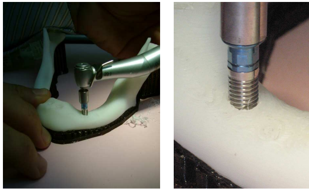
Figura 4: generación de la rosca e inserción del implante
