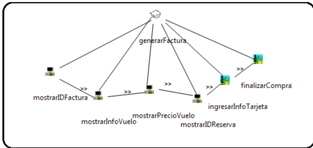
Figura 2.4: Modelo de Tareas. Presentación Propia del autor
