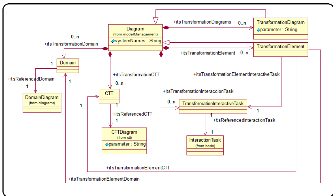
Figura A.13: Modelo de Transformación de Elementos
