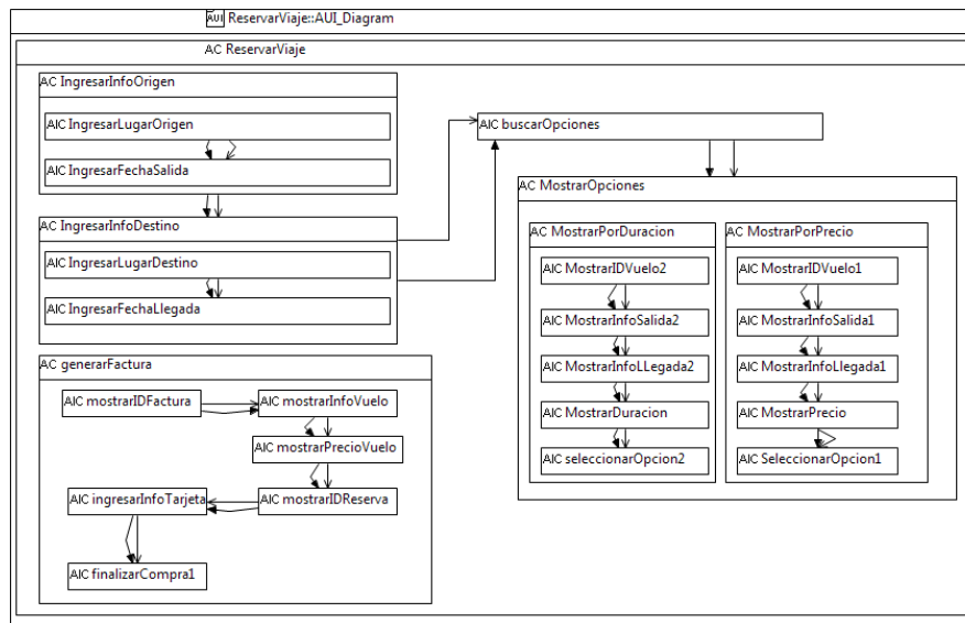
Figura 5.5: Interfaz Abstracta de Usuario: ReservarViaje .
