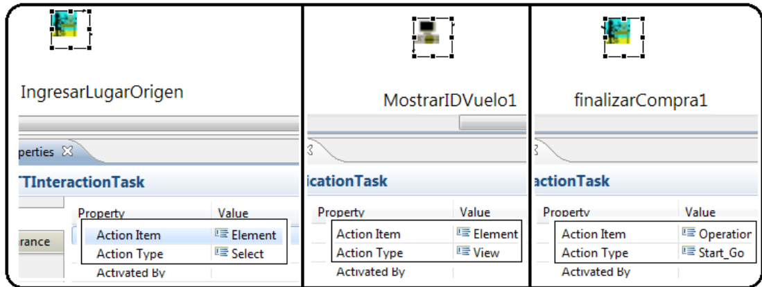
Figura 5.4: Configuración de tareas del modelo CTT de acuerdo a la acción que llevan a cabo sobre el modelo de dominio.
