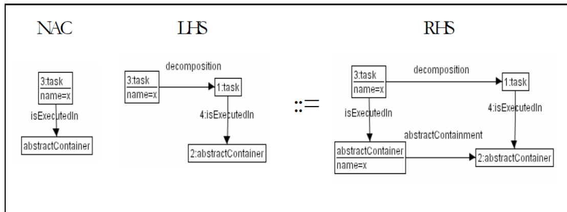
Figura 4.11: Creación de un contenedor abstracto AC derivado de la estructura del modelo de tareas.
