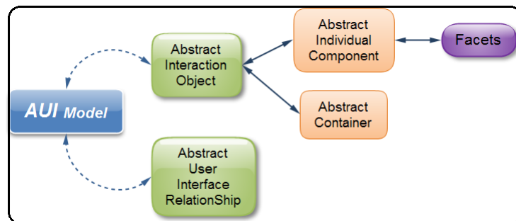
Figura 2.7: Modelo AUI. Presentación propia del autor.
