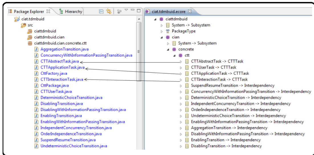
Figura 4.6: Correspondencia entre .genmodel y código generado automáticamente
