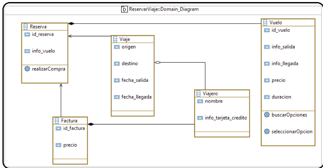
Figura 5.2: Representación del Dominio para caso de estudio propuesto
