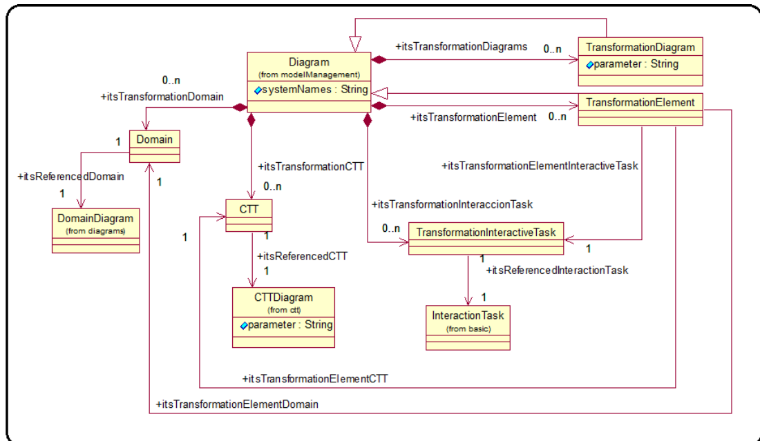
Figura 4.4: Modelo de Transformación.
