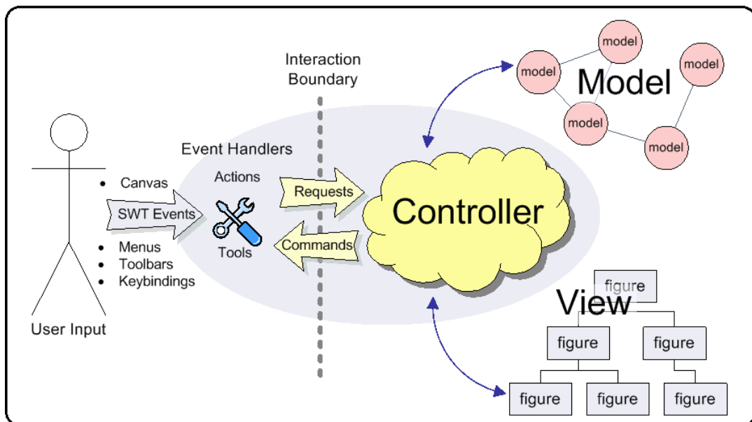
Figura 3.5: Patrón MVC. Tomado de [76]
