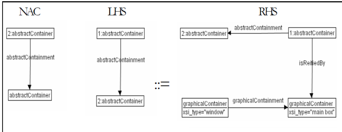
Figura 4.19: Creación de ventana a partir de relaciones de contención.
