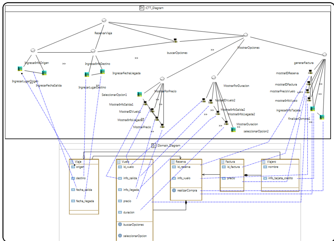
Figura 5.3: Modelo de Mapping para la tarea ReservarViaje
