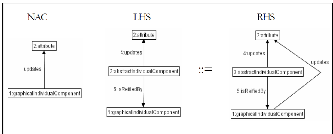
Figura 4.25: Creación de la relación 'Updates'.
