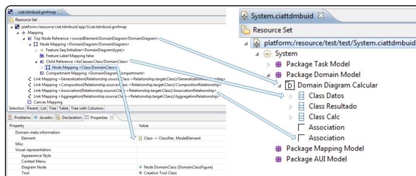
Figura 4.10: Definición Mapping para ciat.tdmbuid
