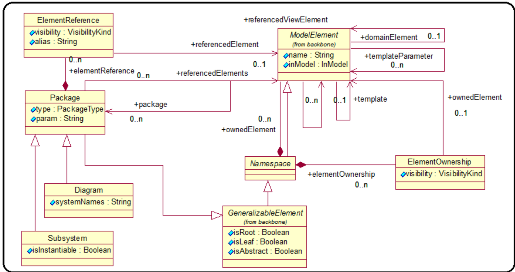
Figura A.2: Gestión de Diagramas. Paquete Model Management .
