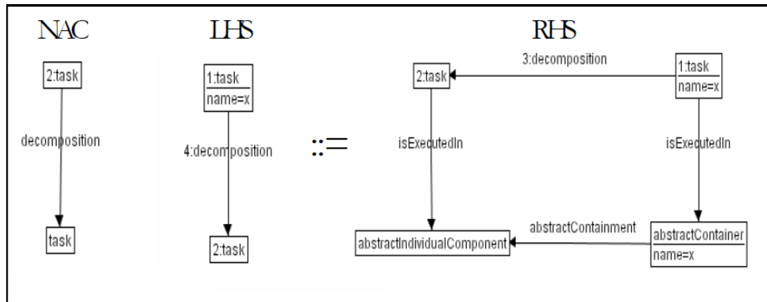
Figura 4.12: Creación de un Componente Individual Abstracto AIC derivado de la estructura del modelo de tareas.
