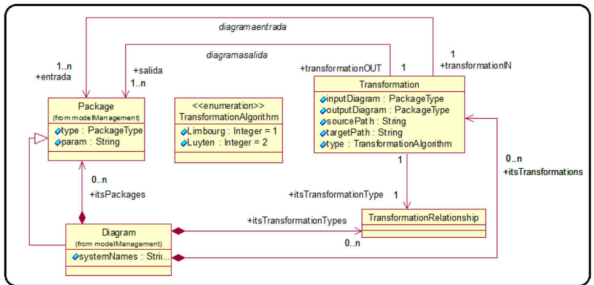
Figura A.12: Modelo de Transformación
