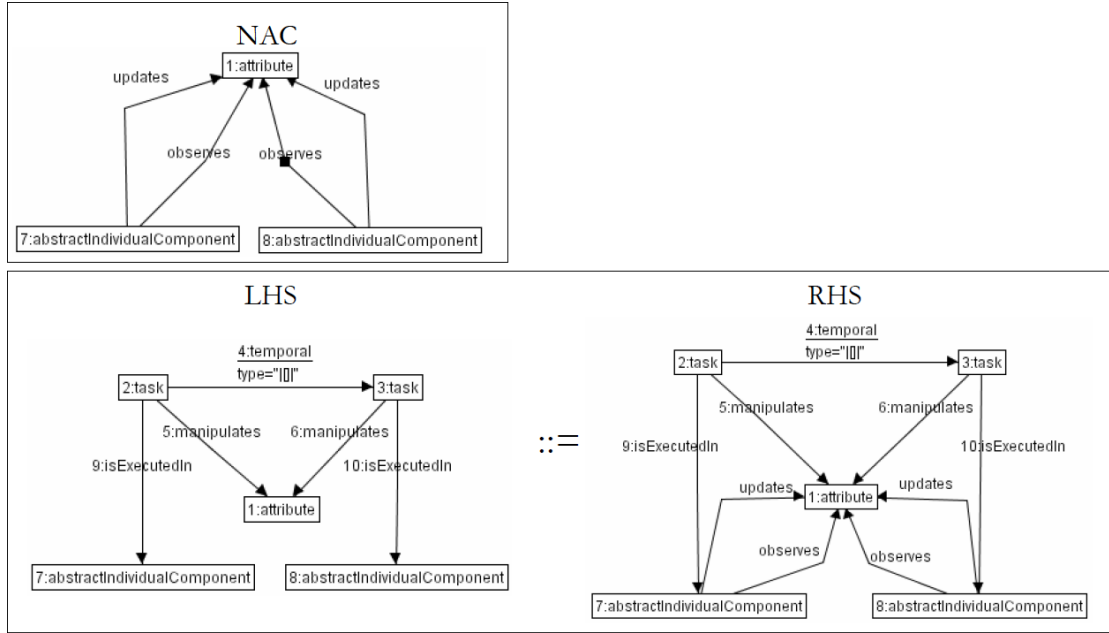
Figura 4.18: Derivación de relaciones Updates y Observes a partir de ConcurrencyConPasoDeInformación \{\square\} .
