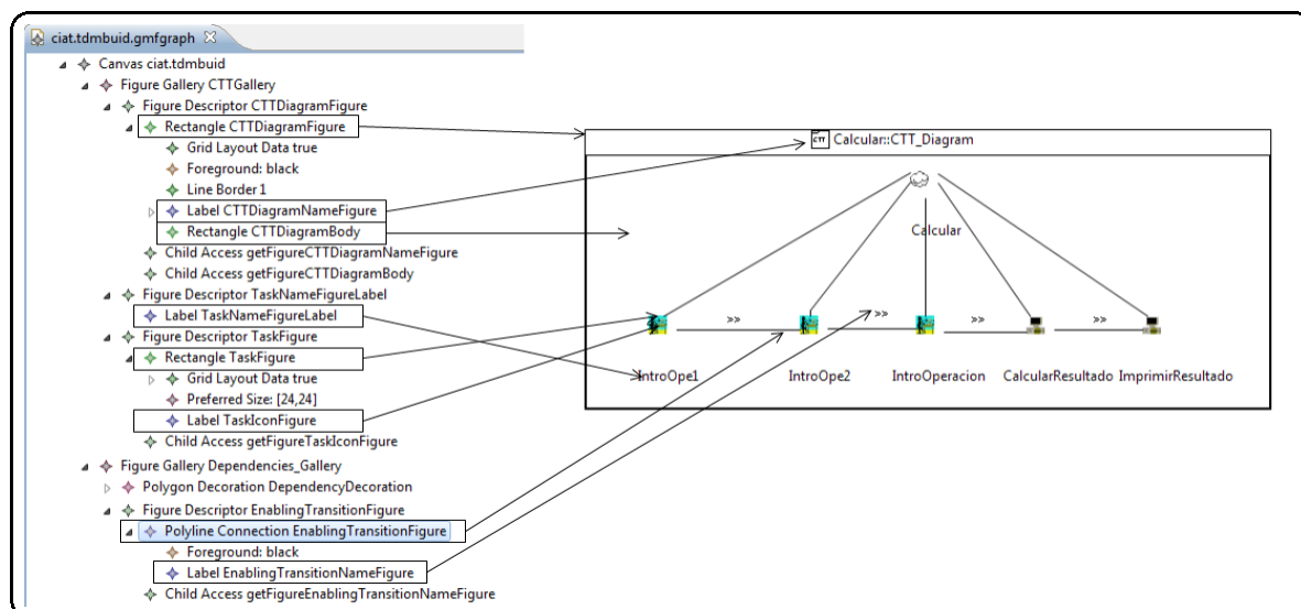
Figura 4.8: Definición Gráfica para el diagrama CTT.
