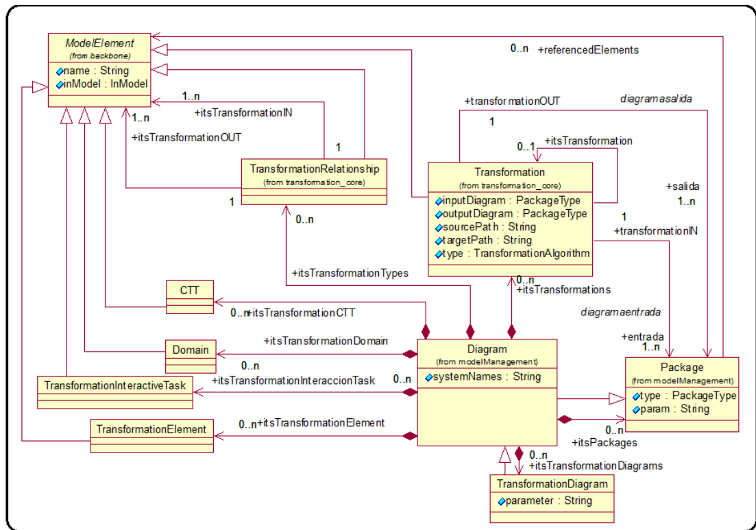
Figura 4.5: Contención de Transformaciones
