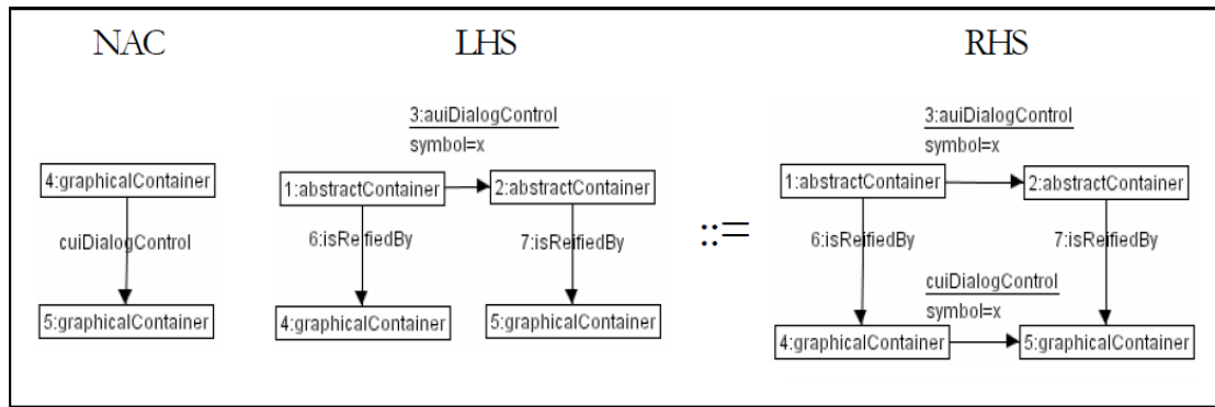
Figura 4.24: Definición del diálogo concreto.
