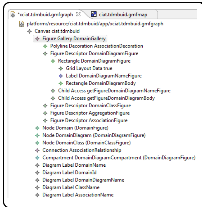
Figura 3.6: Modelo de Definición Gráfica para ciat.tdmdbuid
