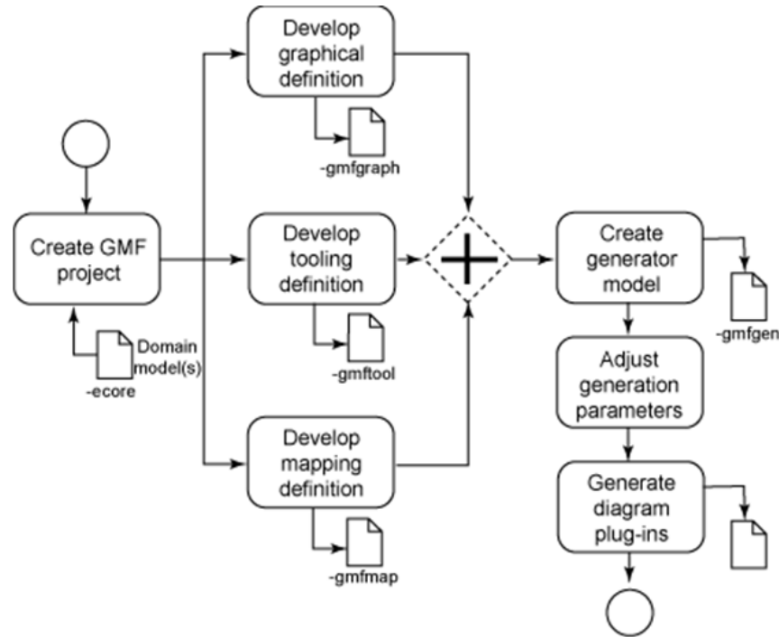
Figura 4.1: Metodología de desarrollo para la construcción de CIAT.TDMBUID . Tomado de [81]
