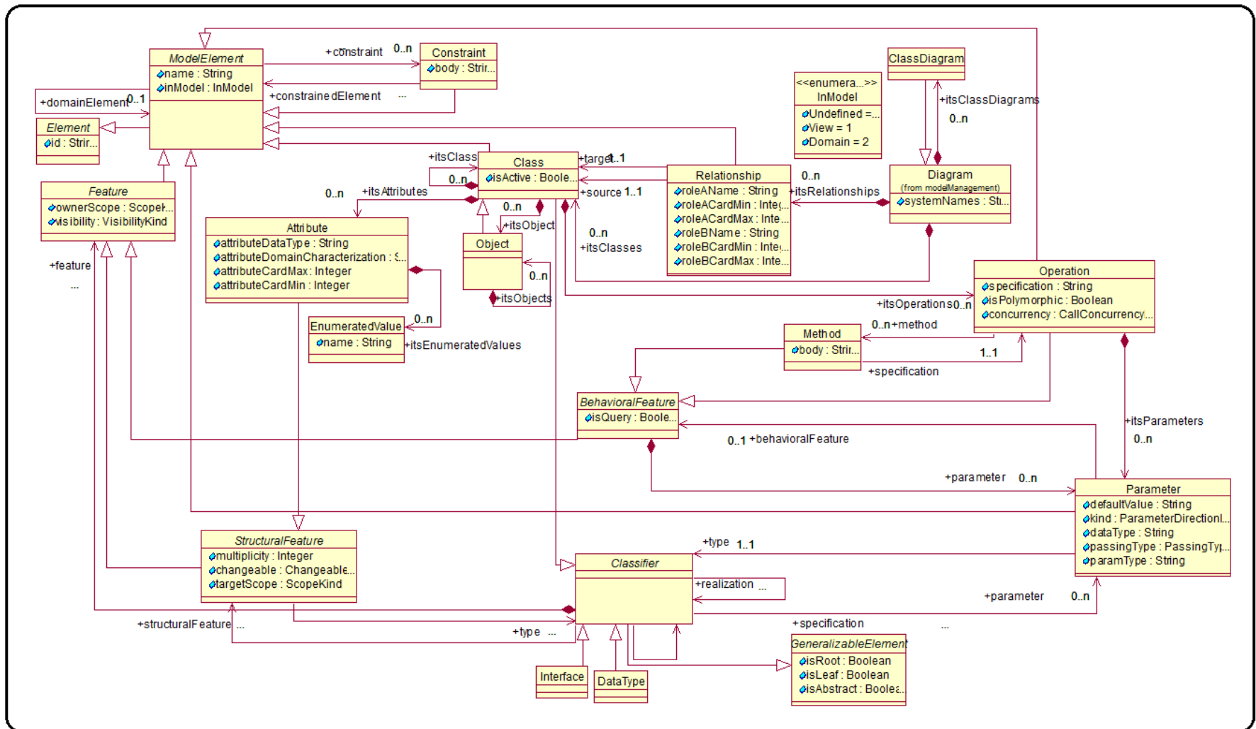
Figura A.3: Paquete backbone . Modelo de Dominio para el editor implementado
