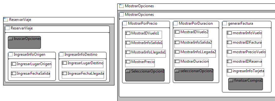
Figura 5.6: Interfaz Concreta de Usuario: ReservarViaje .
