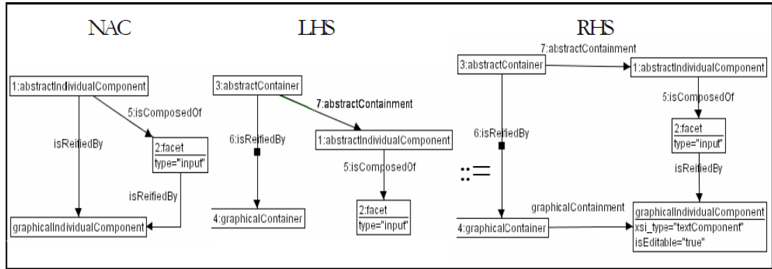
Figura 4.21: Creación de componentes gráficos a partir de sus facets.
