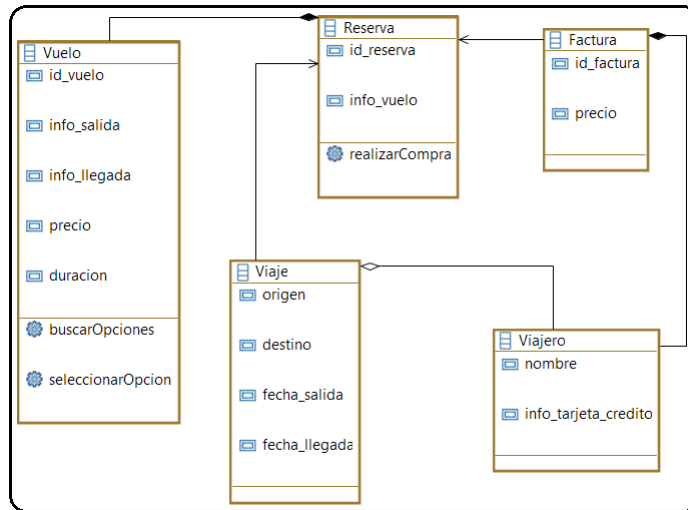
Figura 2.5: Modelo de Dominio. Presentación propia del autor.
