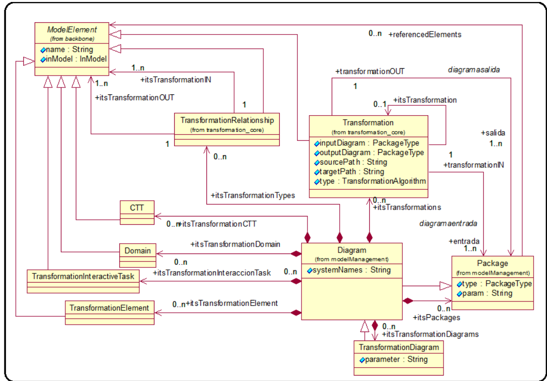
Figura A.11: Modelo de Contención para Transformaciones
