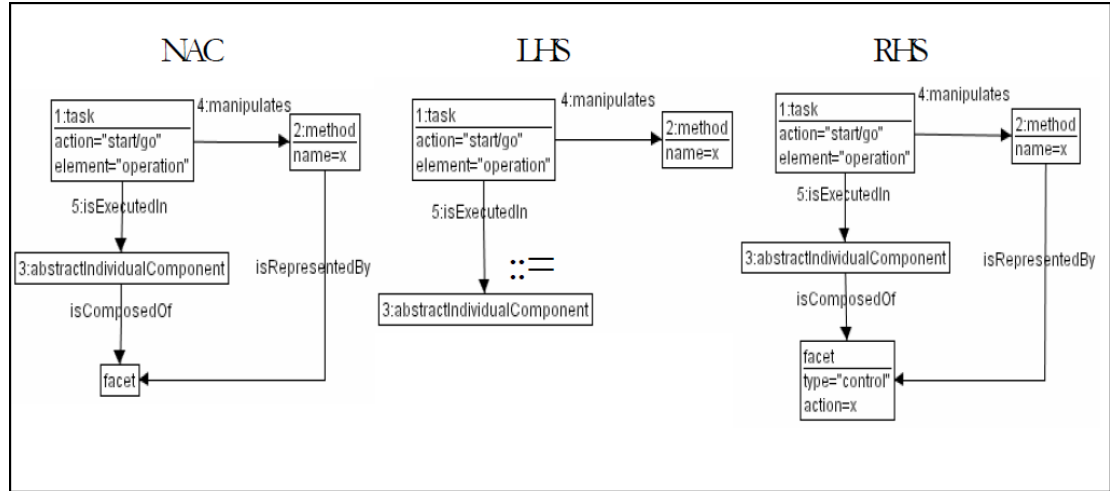
Figura 4.13: Creación de Facets para AICs derivado de la estructura del tipo de acción de tarea.
