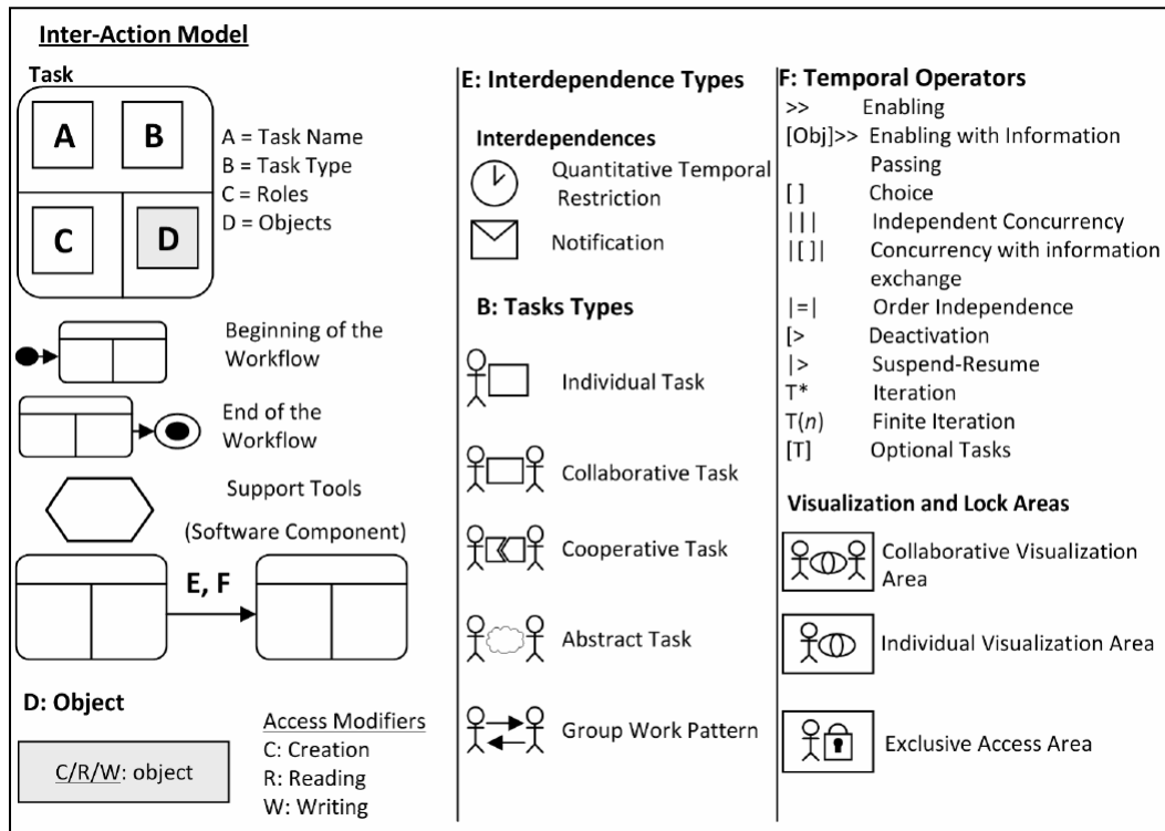
Figura 2.9: Elementos de CIAN. Tomado de [26]
