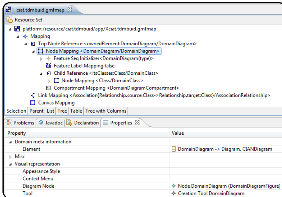
Figura 3.9: Ejemplo mapeo para diagrama de Dominio
