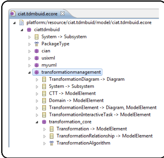
Figura A.10: Modelo de Gestión de Transformaciones para CIAT.TDMBUID
