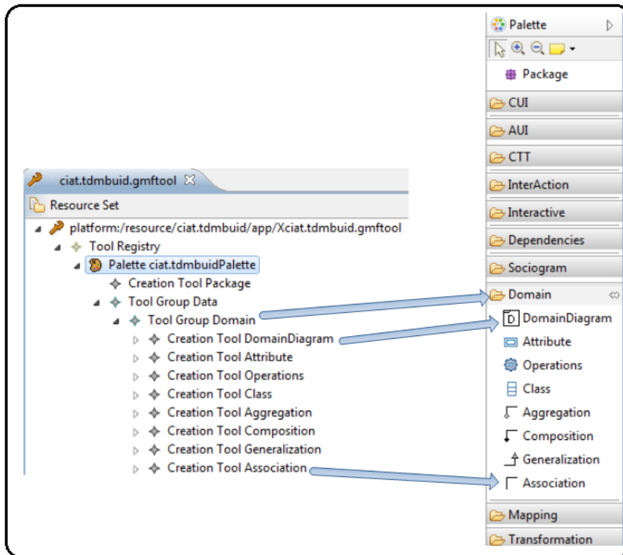
Figura 4.9: Definición Herramienta para ciat.tdmbuid
