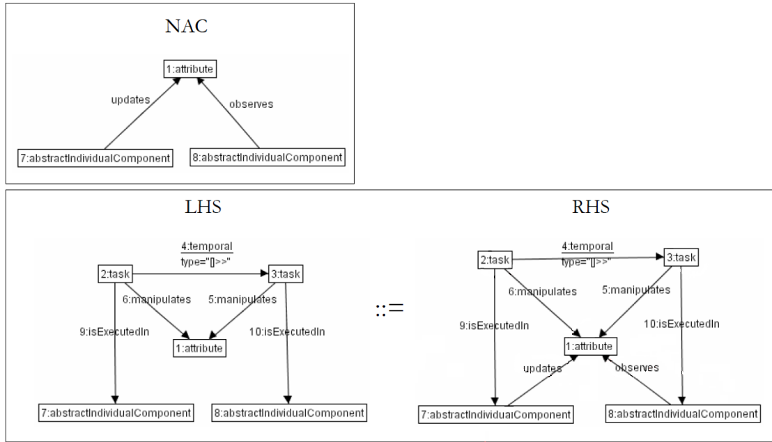
Figura 4.17: Derivación de relaciones Updates y Observes a partir de ActivaciónConPasoDeInformación '[] >>'.
