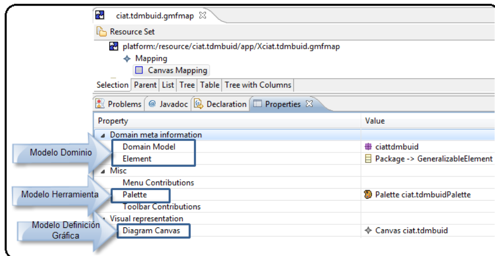
Figura 3.8: Modelo de Mapeo para ciat.tdmbuid
