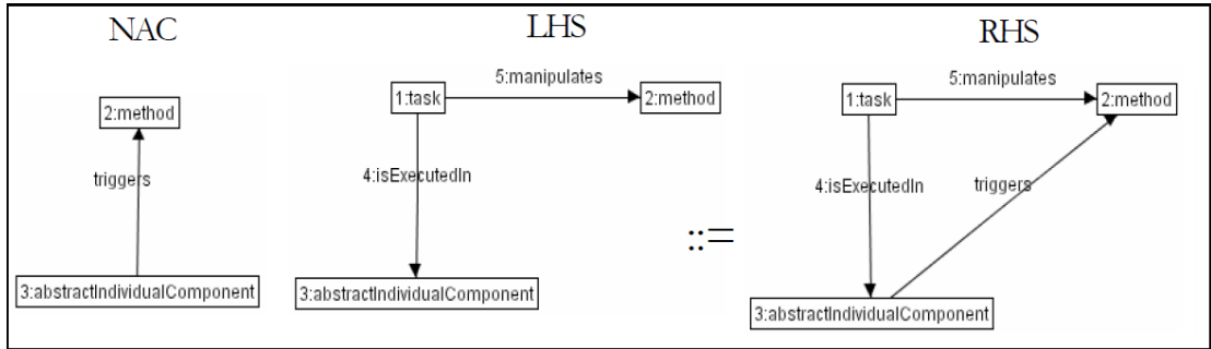
Figura 4.16: Ejecución de método derivado del mapeo entre modelo de tareas y modelo de dominio.
