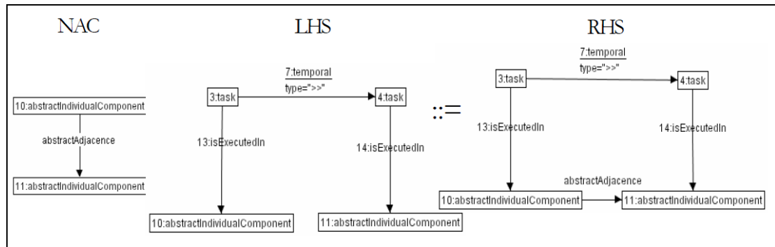
Figura 4.14: Creación de adyacencia entre AIOs derivada de relaciones temporales de secuencialización.
