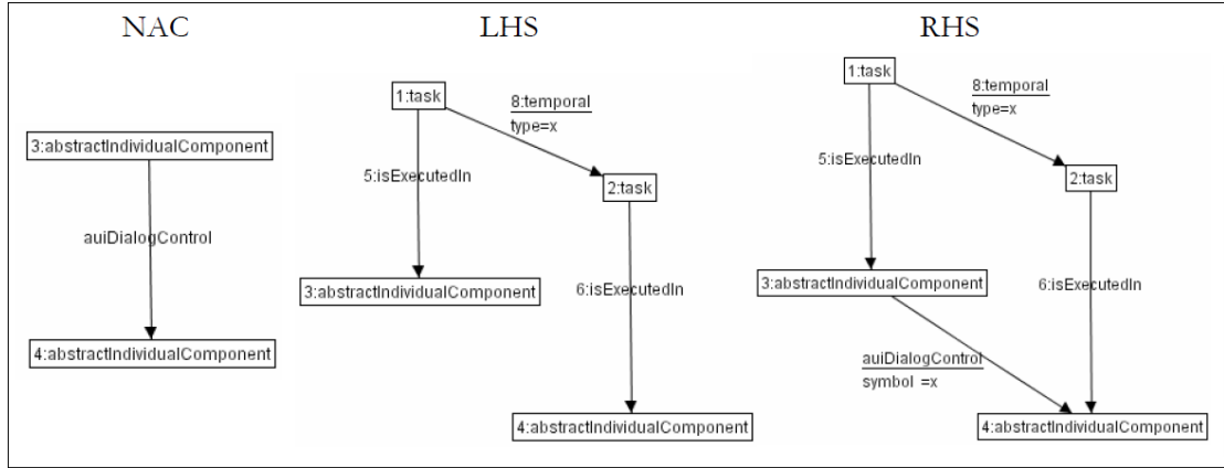
Figura 4.15: Creación de Dialog Control derivado del modelo de tareas.
