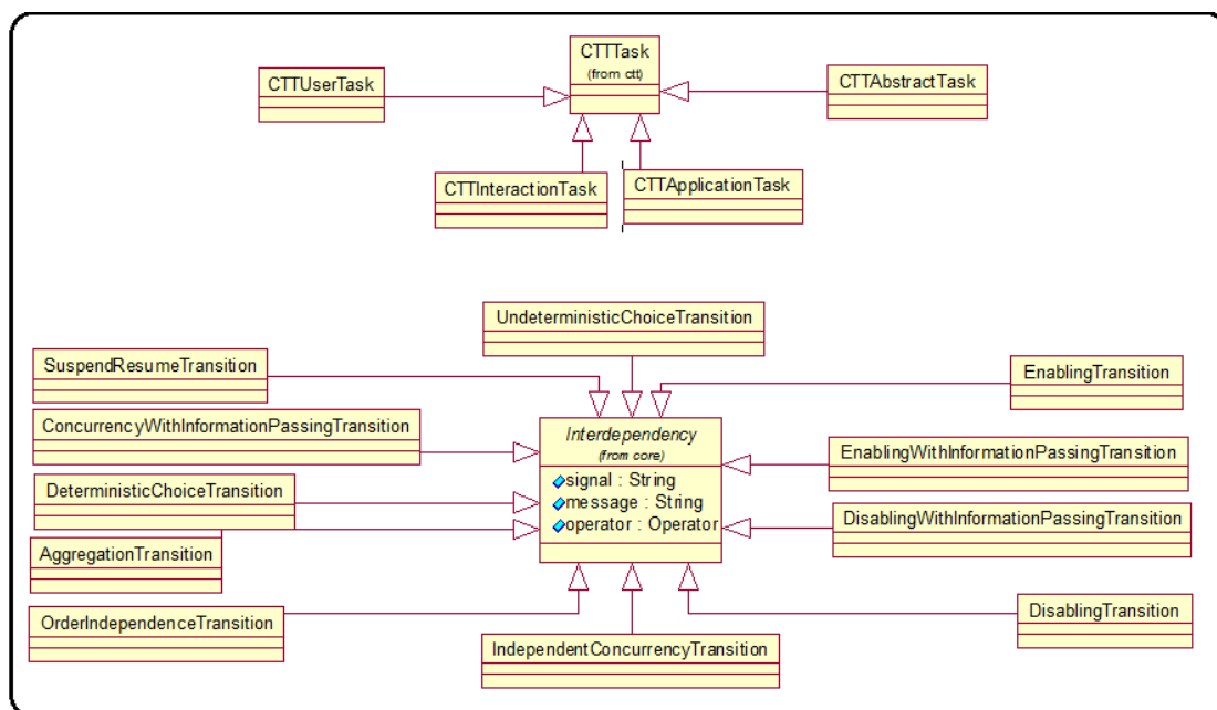
Figura A.6: Tipos de Tareas CTT.
