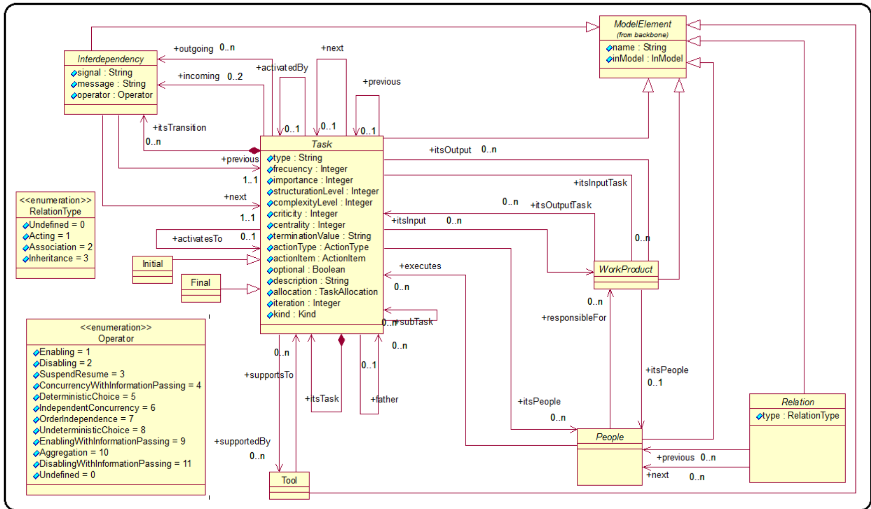
Figura A.4: Paquete CIAN.core
