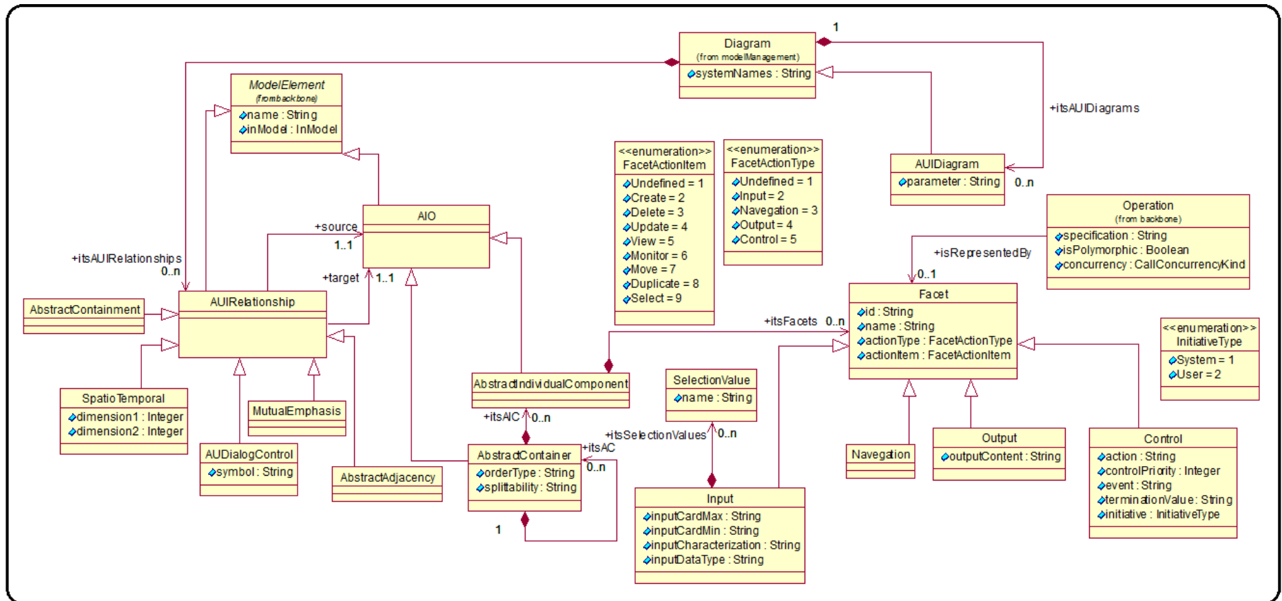
Figura A.7: Modelo AUI para el editor implementado
