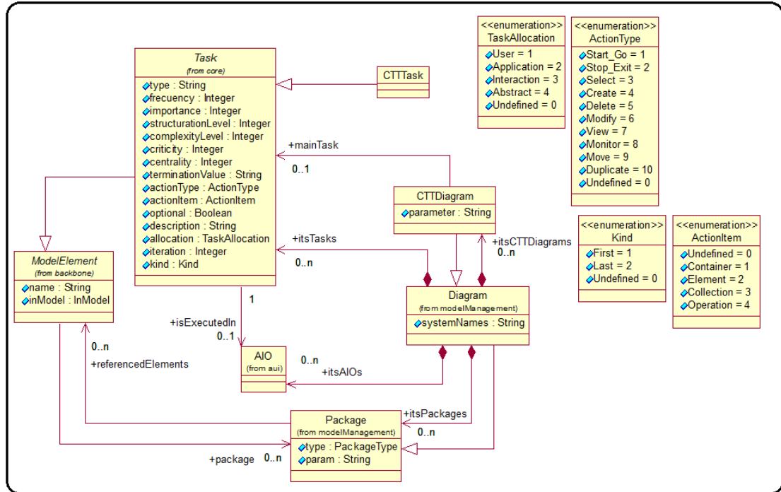
Figura A.5: Paquete CTT.
