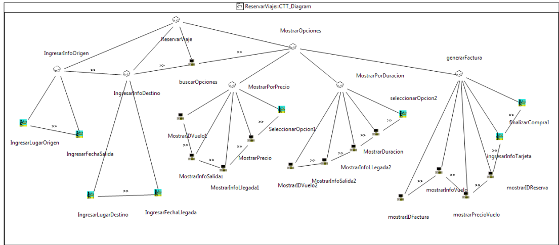
Figura 5.1: Diagrama CTT para tarea ReservarViaje
