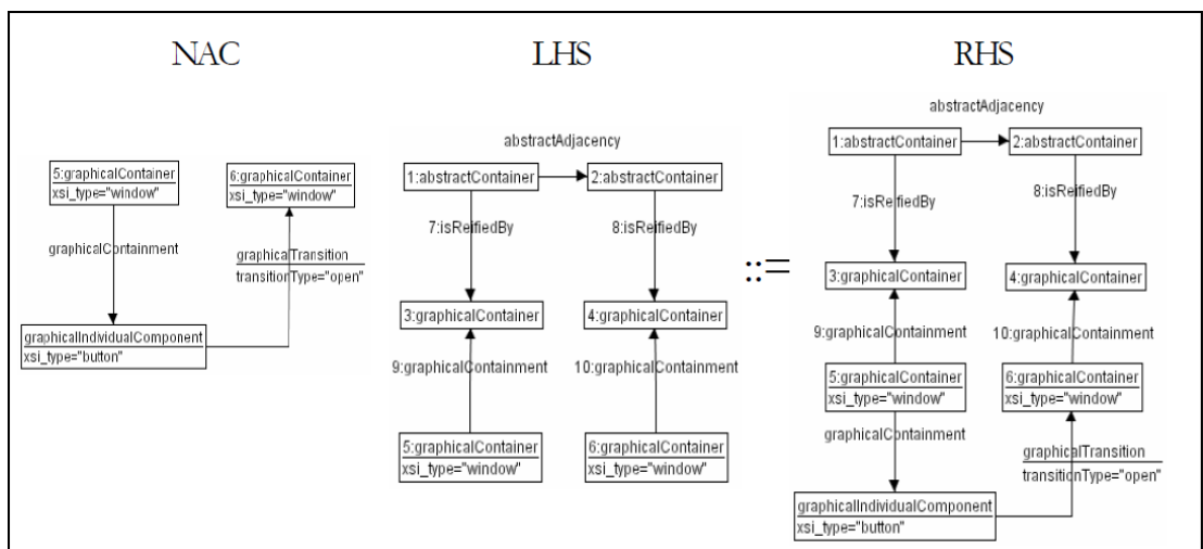
Figura 4.23: Definición de la navegación en distintos contenedores.
