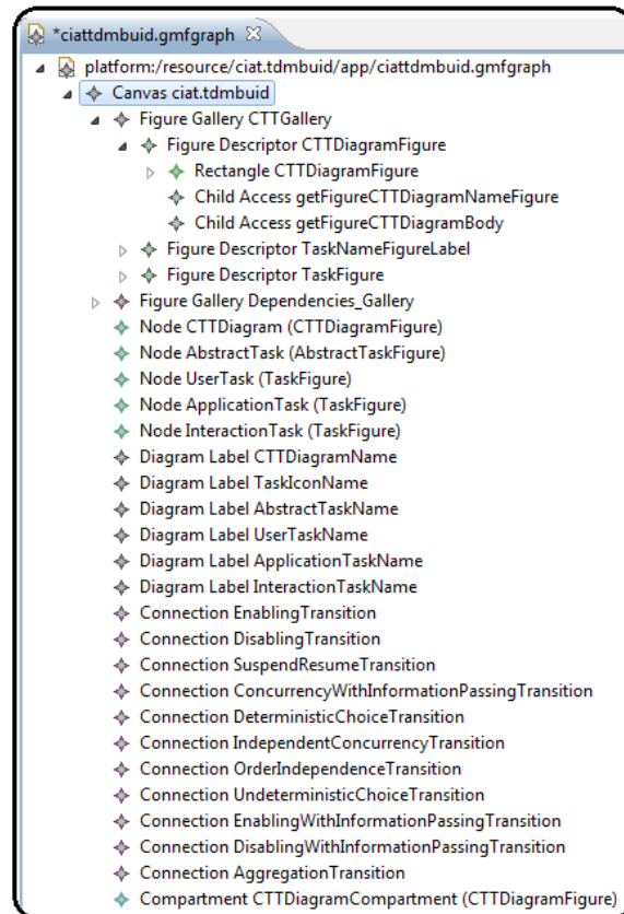
Figura 4.7: Definición gráfica para ciat.tdmbuid
