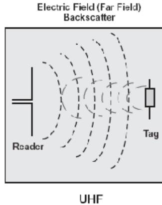
FIGURA 4 - EFECTO BACKSCATTER
