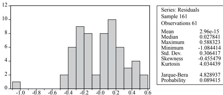
Gráfico 1. Normalidad
