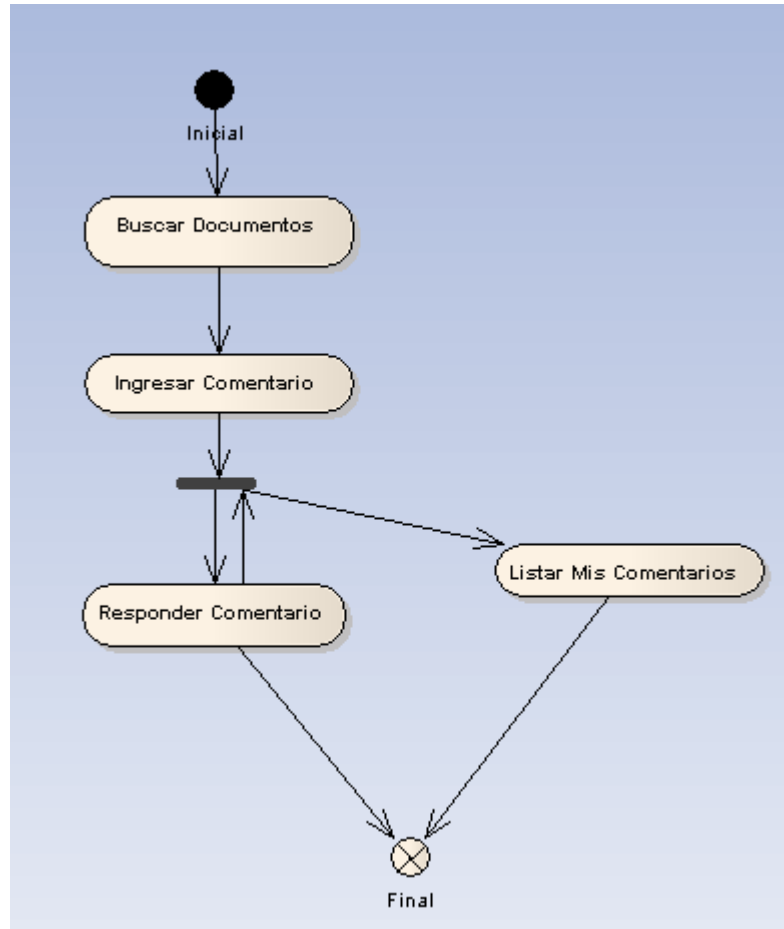
FIGURA 11. DIAGRAMA DE ACTIVIDADES MODULO DE COMENTARIOS.
