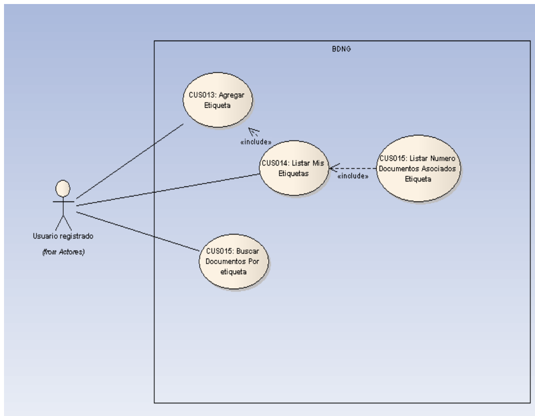
FIGURA 12. DIAGRAMA DE CASOS DE USO DEL MODULO DE ETIQUETAMIENTO.
