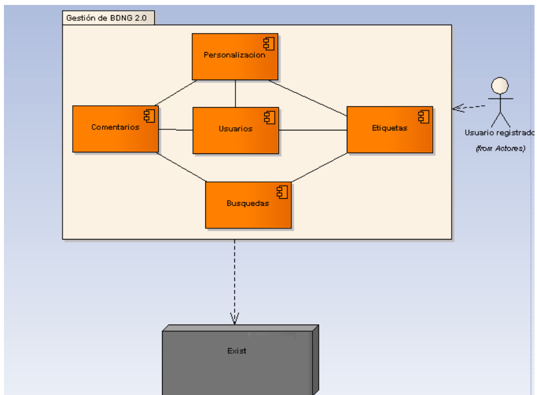
FIGURA 7. ARQUITECTURA ESPECÍFICA DE BDNG 2.0
