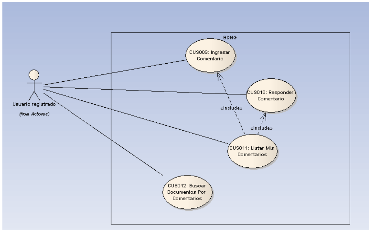
FIGURA 11. DIAGRAMA CASOS DE USO MODULO COMENTARIOS.
