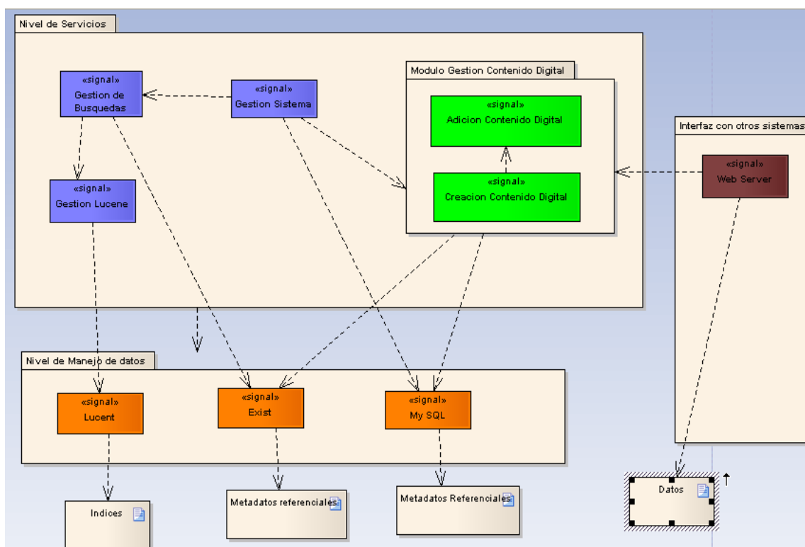
FIGURA 5. ARQUITECTURA DE BDNG ACTUAL
