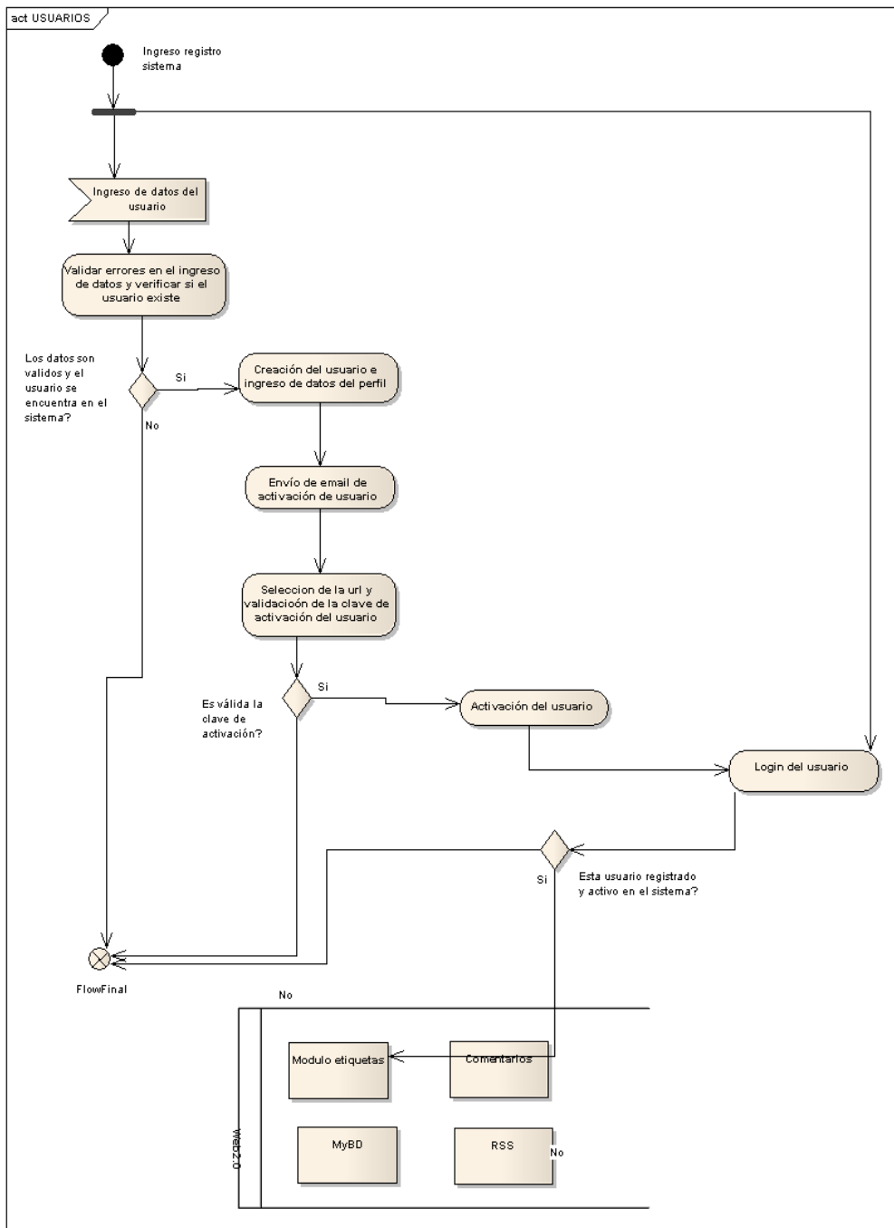
FIGURA 10. DIAGRAMA DE ACTIVIDADES DEL MODULO DE USUARIOS.
