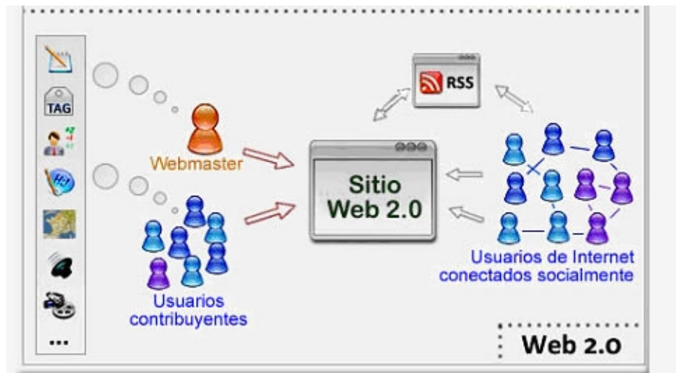
FIGURA 2. CONCEPTO WEB 2.0
