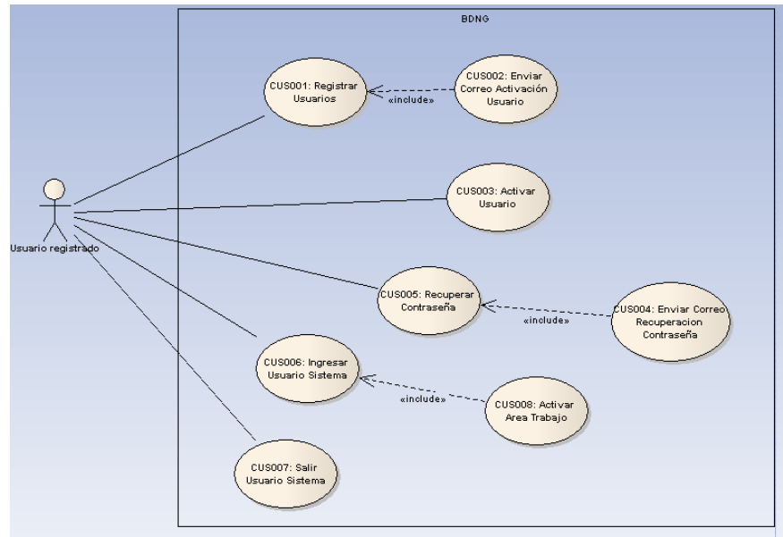
FIGURA 10. DIAGRAMA CASOS DE USO GENERALES MODULO DE USUARIOS.
