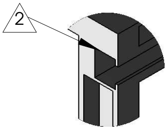
Detalle B. Riel diada Escala 1:10
