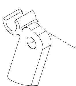
Detalle A Soporte Escala 1:5
