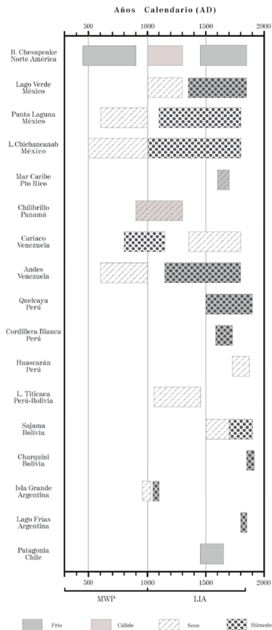
Figura 4. Representación de las condiciones paleoclimáticas y periodos correspondientes al Periodo Cálido Medieval (MWP) y la Pequeña Edad de Hielo (LIA) para los registros mencionados en el texto. Se muestran siete interpretaciones paleoclimáticas correspondientes a clima frío, cálido, seco, húmedo, cálido-seco, frío-seco y frío-húmedo. (Compilado de: Thompson et al. , 1986; Rull et al. , 1987; Hodell et al. , 1995; Curtis et al. , 1996; Abbott et al. , 1997; Winter et al. , 2000; Haug et al. , 2001; Lachniet et al. , 2001; Rabatel et al. , 2001; Watanabe et al. , 2001; Cronin et al. , 2003; Hodell et al. , 2005; Liu et al. , 2005; Polissar et al. , 2006a; Ariztegui et al. , 2007; Harrison et al. , 2007; Lozano-García et al. , 2007; Solomina et al. , 2007).
