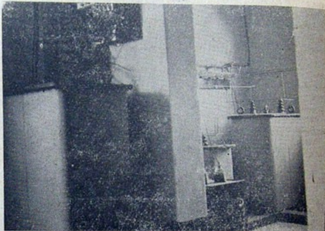
AGRUPADOS aparecen los transformadores de PODER y de MODULACION, partes principales del equipo transmisor: de la calidad de estas piezas depende en un todo la fidelidad, limpidez y tono de la transmisión; por ello para los equipos de La Voz de Antioquia se hizo especial elección de lo mejor que hasta la fecha se fabrica en Estados Unidos.
