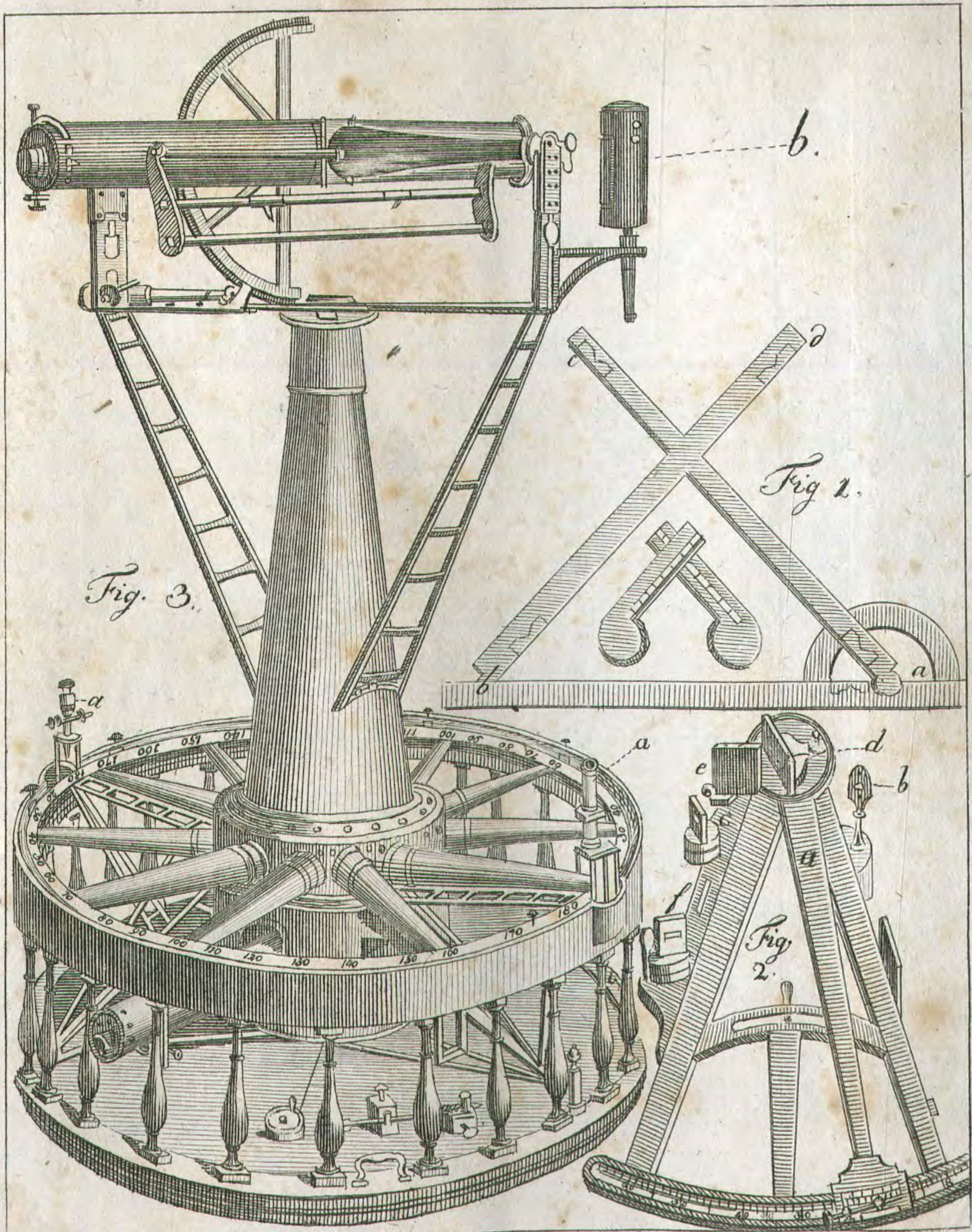
1. Das Triquetrum, 2. der Sextant, 3. das grosse Theodelit.
