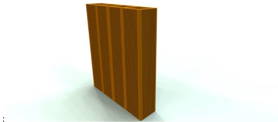
Figura 4. Ladrillo de gran formato a fabricar. Medidas nominales: 10 cm de ancho x 40 cm de alto x 40 cm de largo. Peso estimado cocido: 11Kg. Fuente: Archivo Larillera San Cristóbal S.A.
