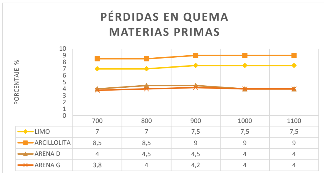
Gráfico 6. Porcentaje de pérdida en la quema de las materias primas analizadas a diferentes temperaturas de cocción.
