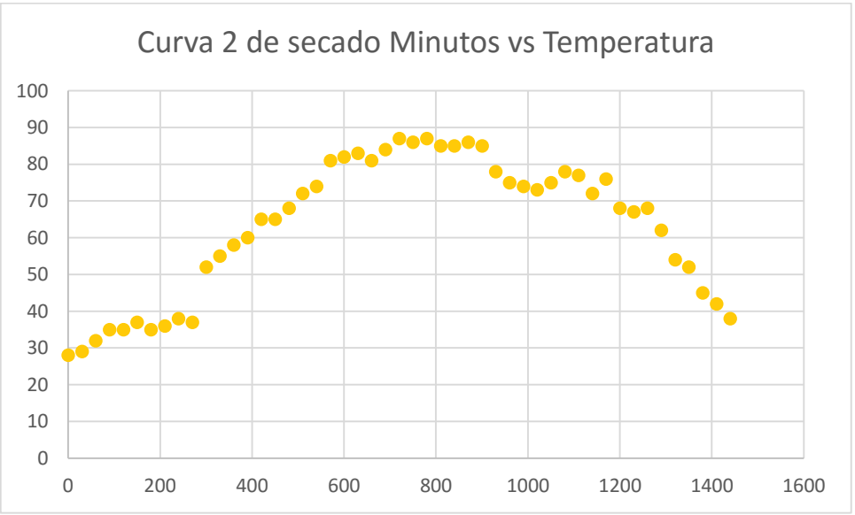
Gráfico 14. Curva de secado 2.
