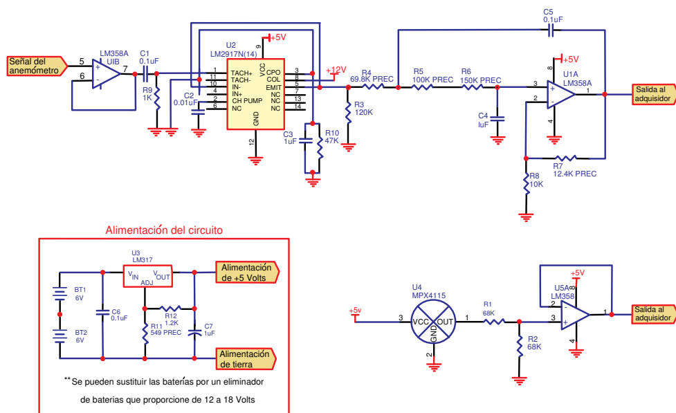
Figura 3: Diagrama general del anemómetro y barómetro
