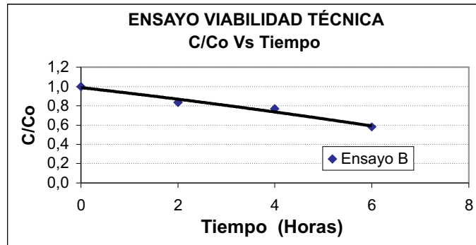
Figura 9: Disminución de DQO vs Tiempo
