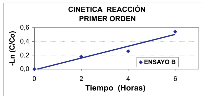
Figura 10: Cinética reacción
