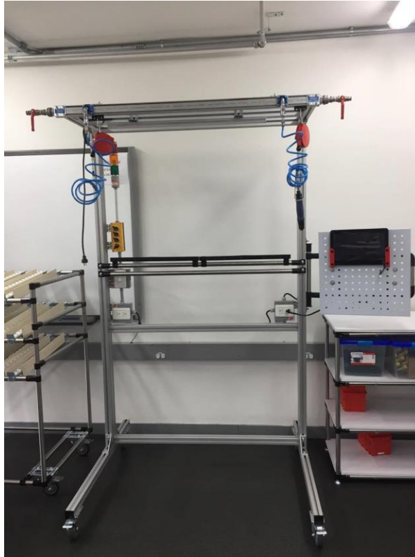
Ilustración 23. Módulo de servicio
