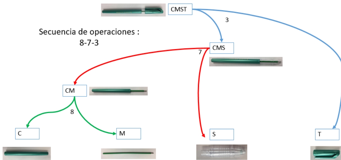
Ilustración 35. Secuencia de ensamble para Lapicero Stabilo Excel. Elaboración propia
