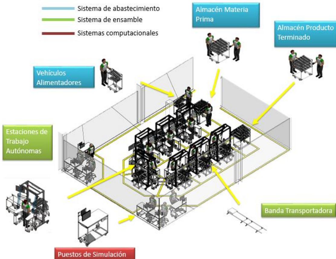
Ilustración 15. Infraestructura física FA Universidad EAFIT
