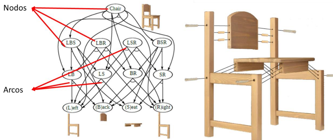
Ilustración 31. Diagrama And/or para Silla (Knepper et al., 2014)
