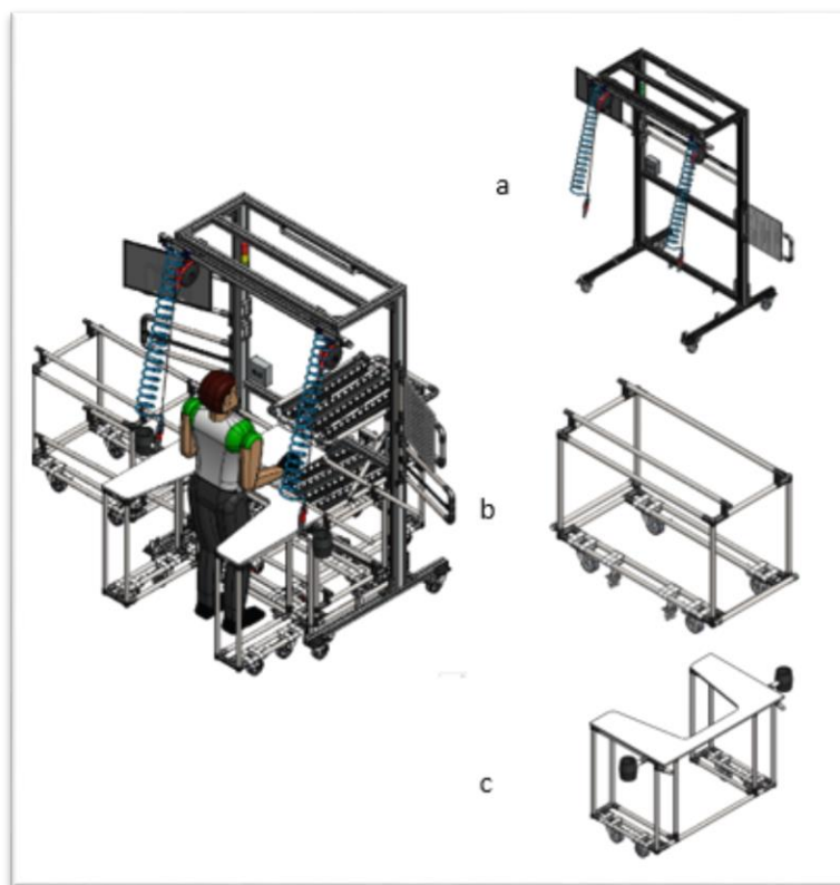
Ilustración 16. Modulo de ensamble a) modulo de servicios, b) modulo de transporte y c) mesa auxiliar.
