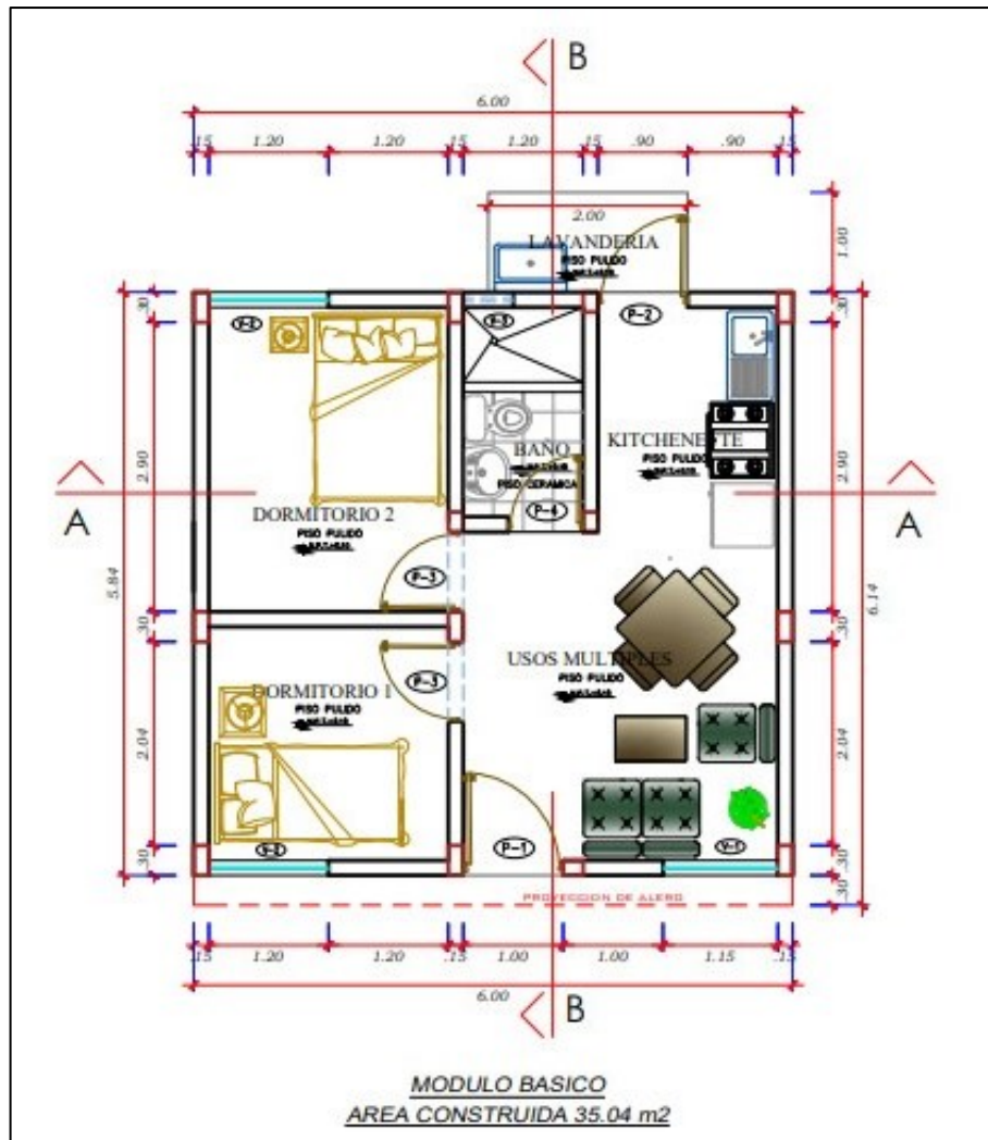
Figura 12. Plano del módulo de 35m 2 , modalidad CSP, del Programa Techo Propio
