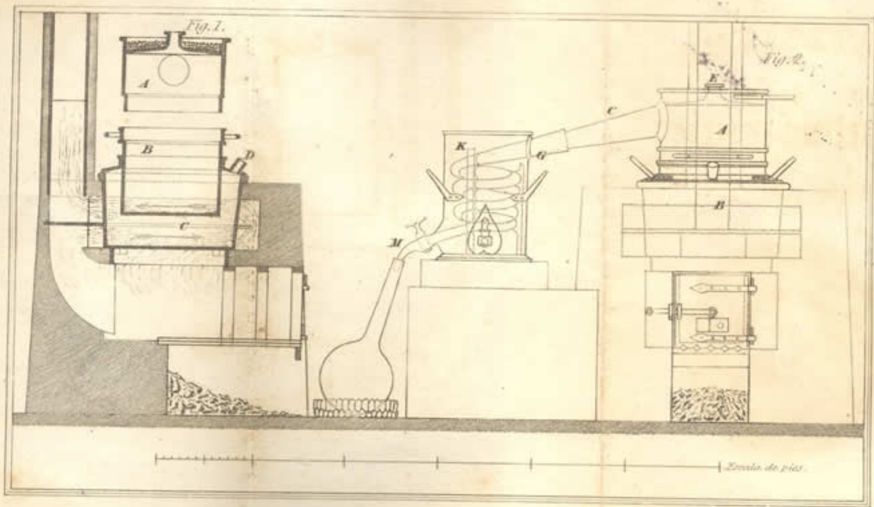
CORTE Y ELEVACION DE UN ALAMBIQUE PERFECCIONADO.
