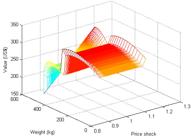
Fig. 4 Value function
