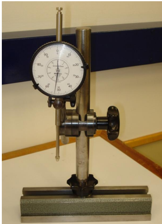
Figura 23. Reloj comparador universidad EAFIT
