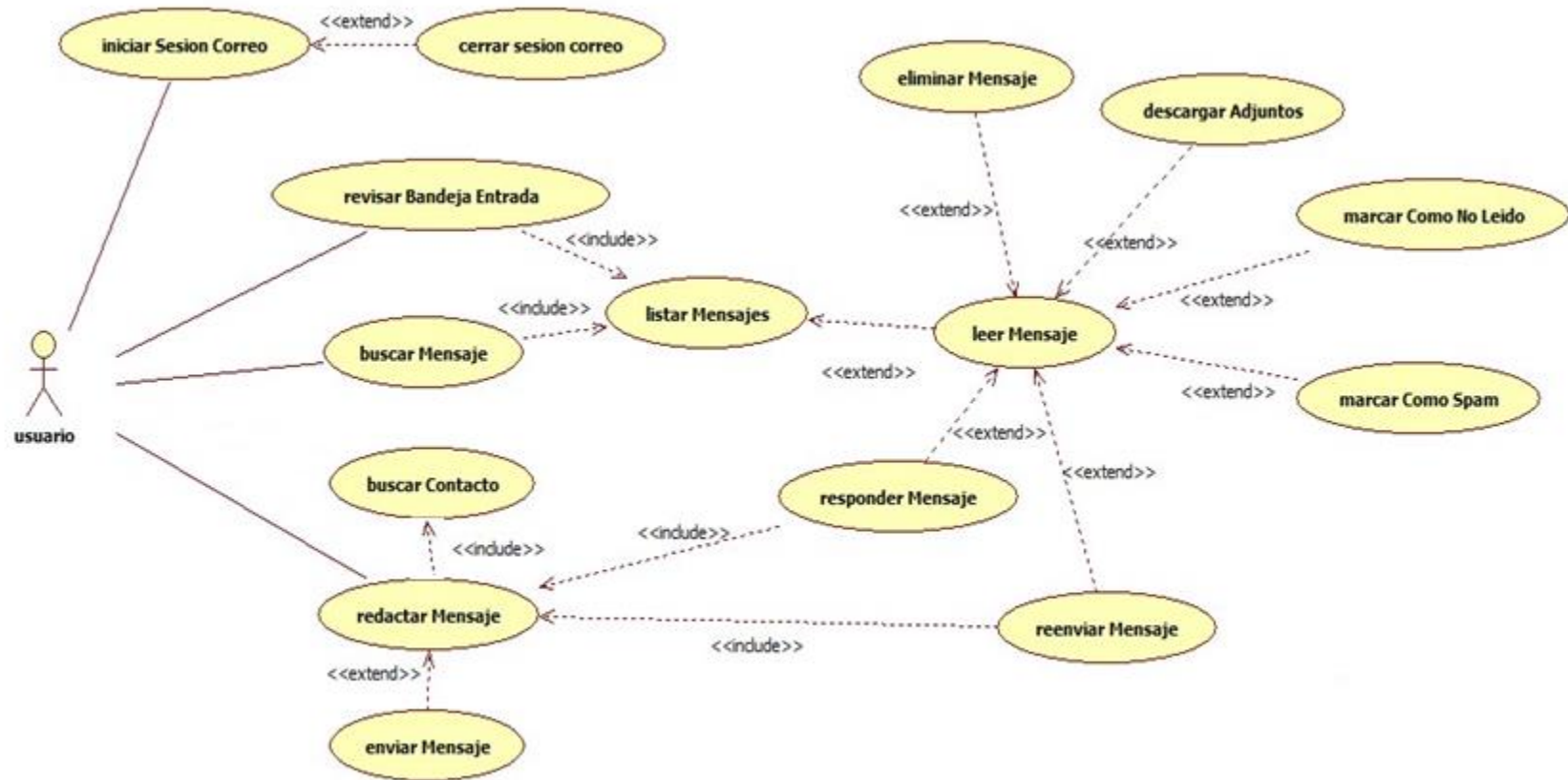
Ilustración 11. Diagrama de Casos de Uso eBlindMail
