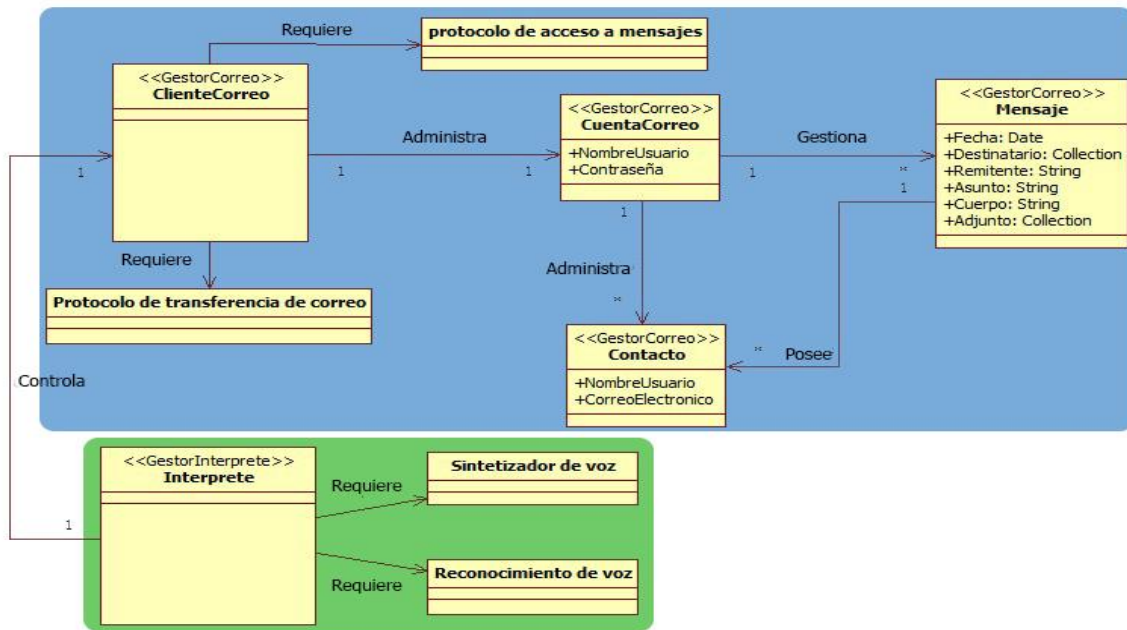
Ilustración 13. Identificación de Componentes
