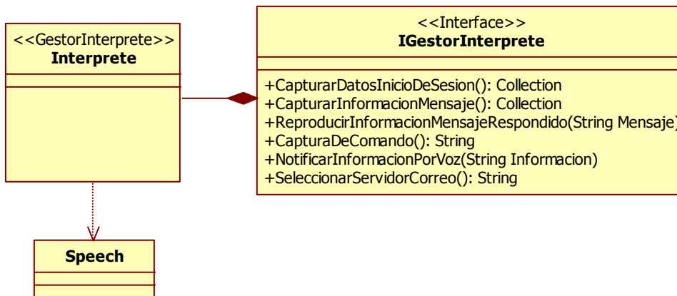
Ilustración 14. Componente GestorInterprete
