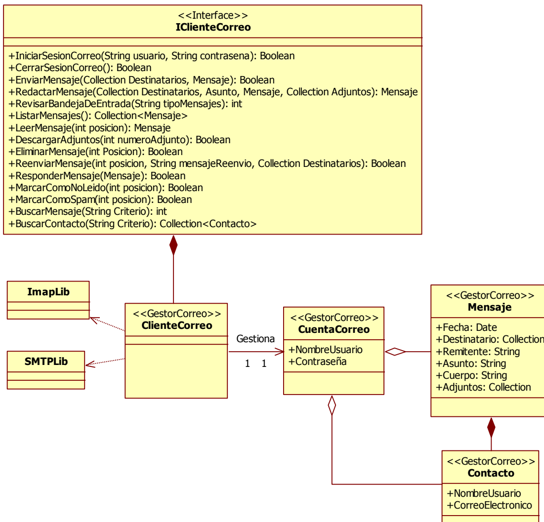
Ilustración 15. Componente GestorCorreo
