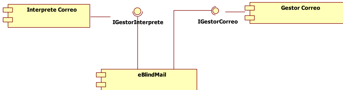
Ilustración 16. Diagrama de componentes
