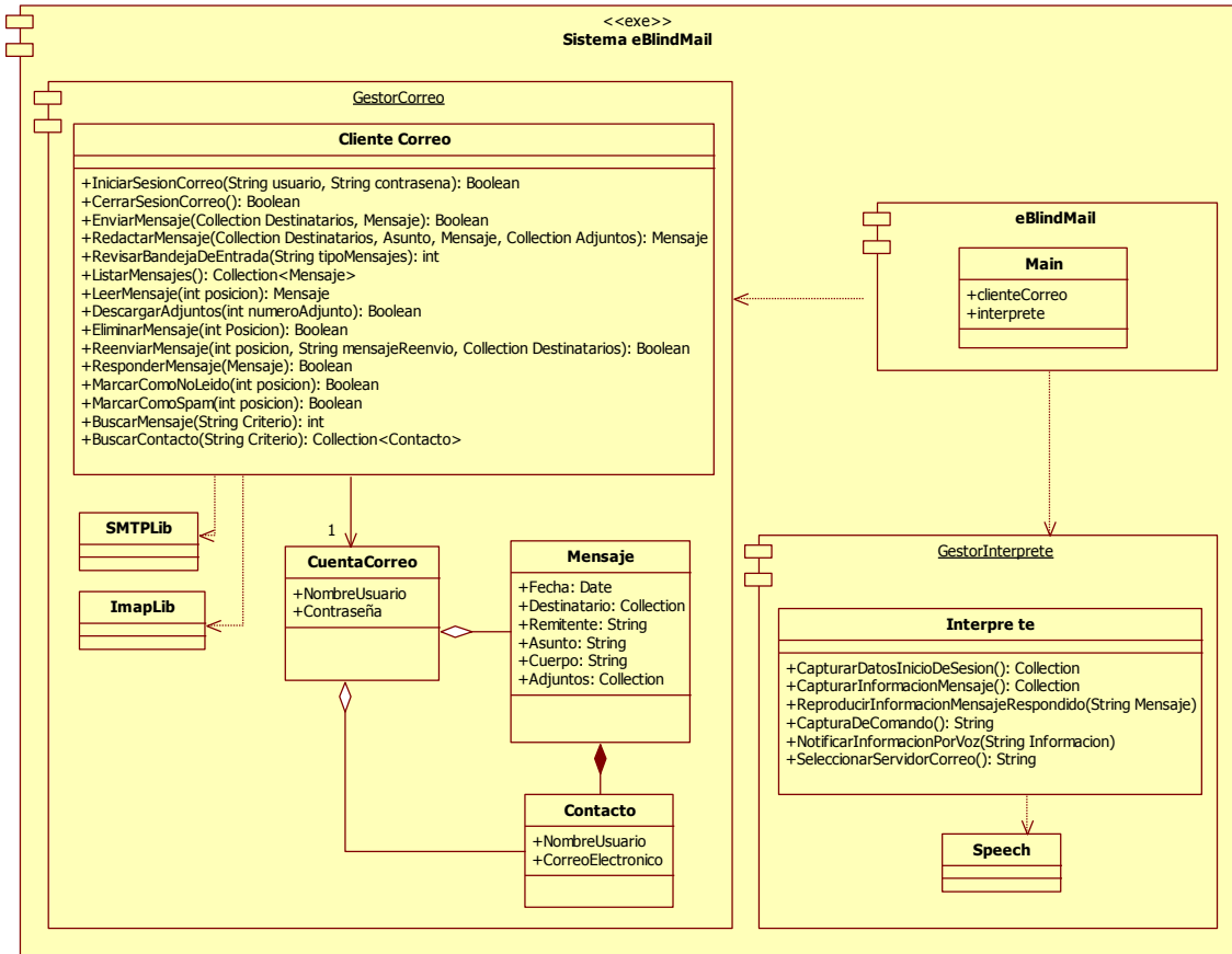
Ilustración 18. Vista de Desarrollo
