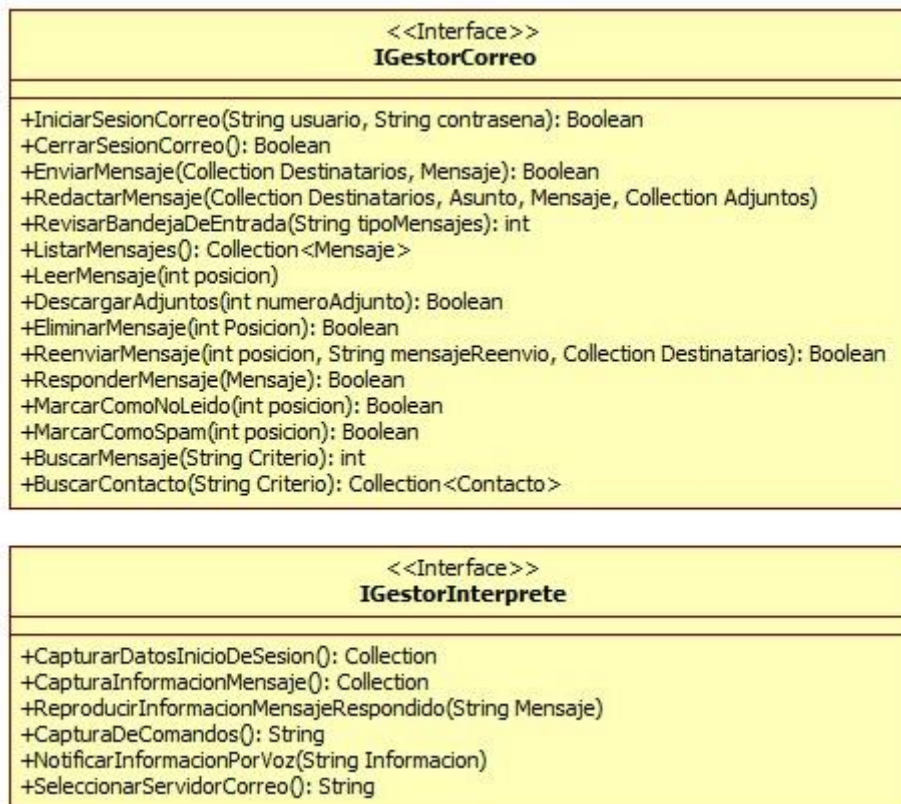
Ilustración 17. Interfaces
