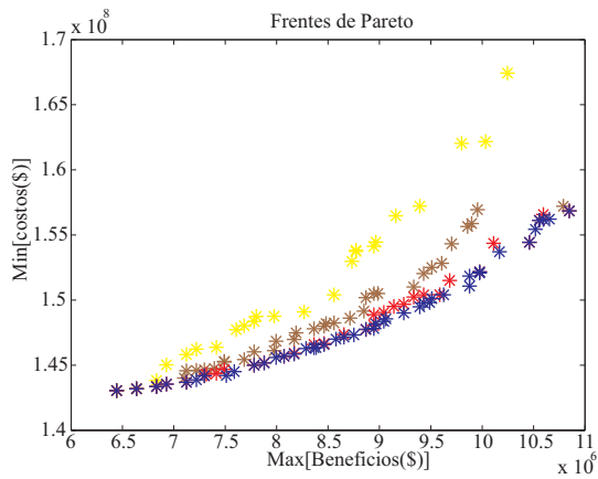
Figura 2: Frentes de Pareto - Conjunto monofásico
