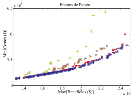
Figura 3: Frentes de Pareto - Conjunto trifásico
