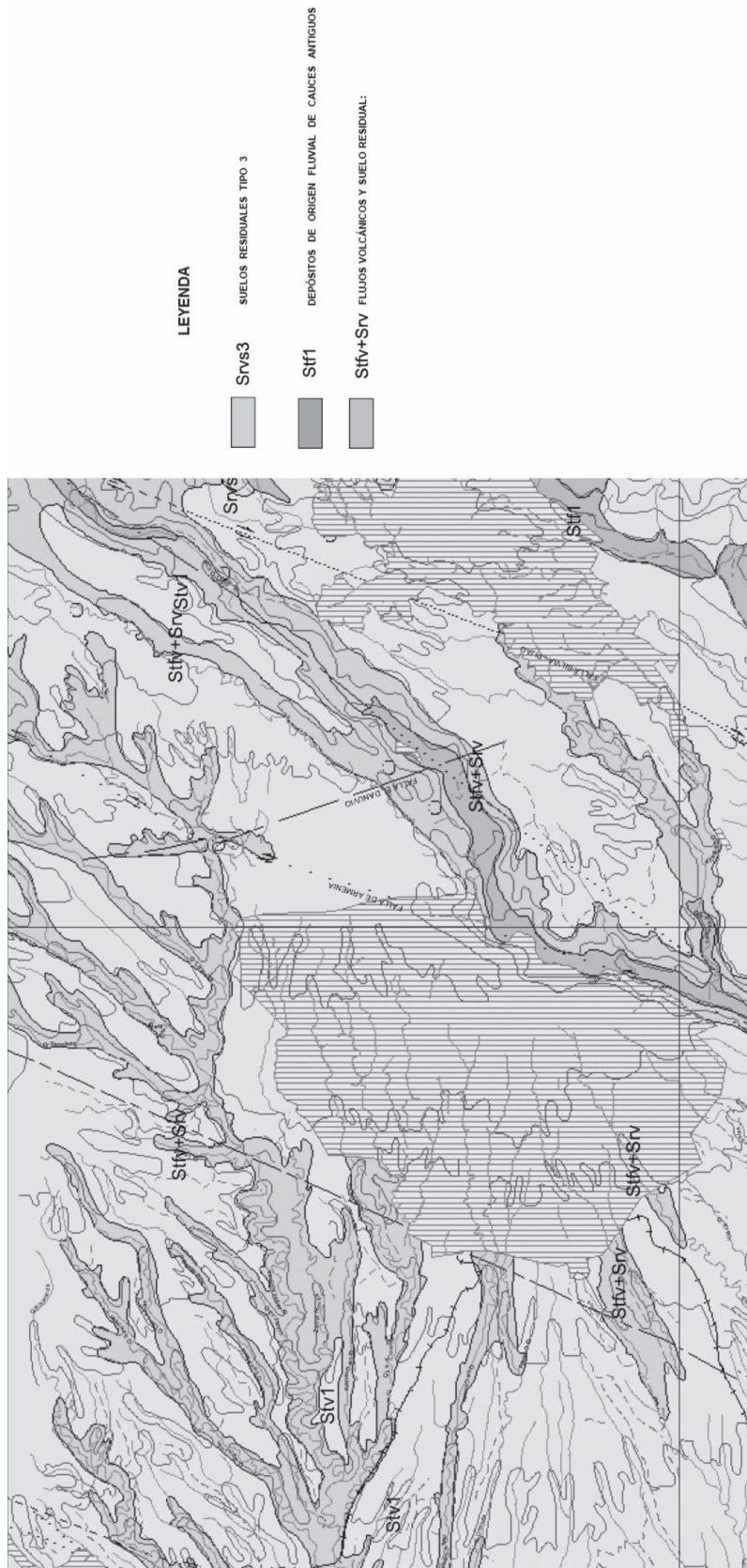
Figura 3. Mapa de la geología superficial de la ciudad de Armenia (tomada de Padilla et al., 2005)
