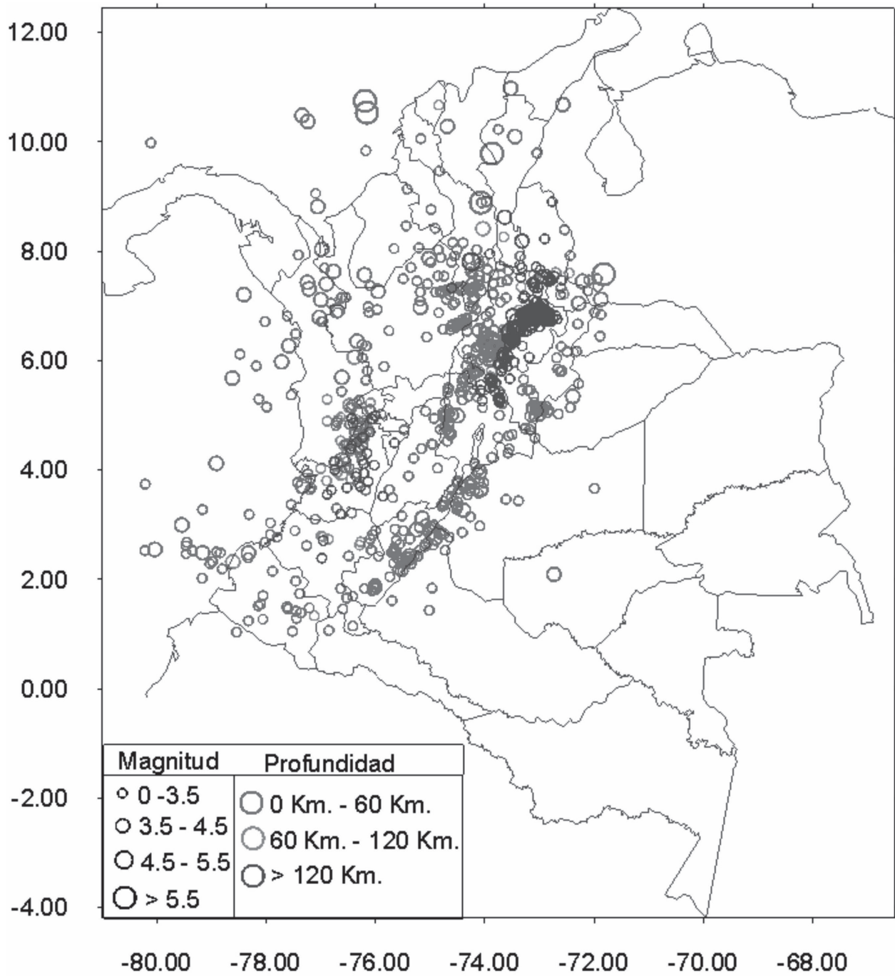
Figura 3. Mapa de sismicidad, por magnitud y profundidad, según la RSNC (Tomado de: www.ingeoimas.com.co )
