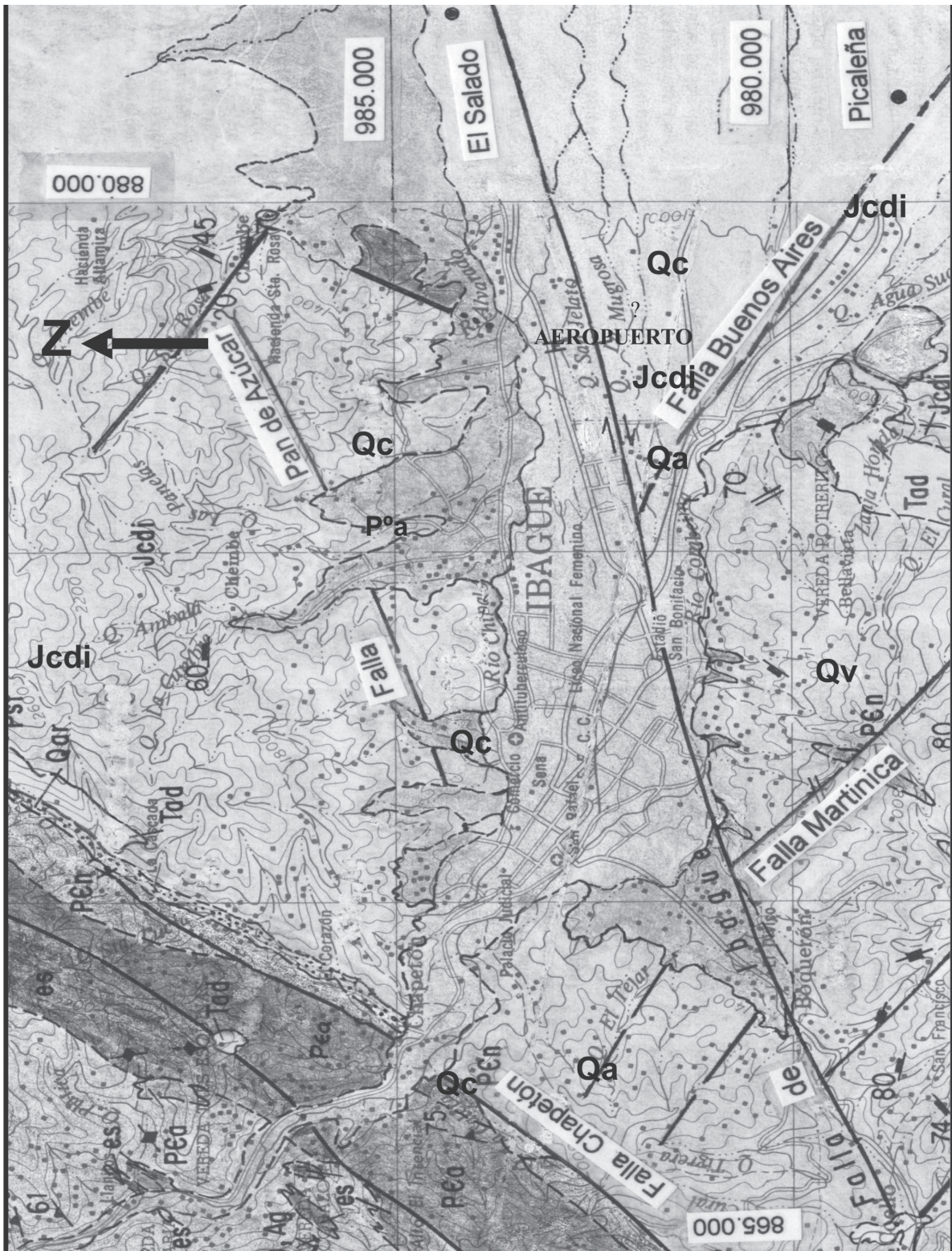
Figura 1. Mapa geológico de Ibagué y alrededores (plancha 244; Mosquera y otros, 1984., plancha 245, Acosta y Ulloa, 1989, con modificaciones)
