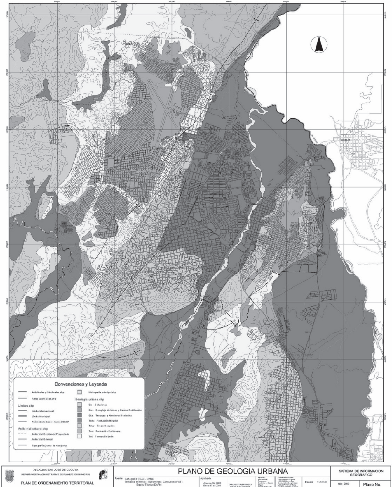
Figura 3. Geología urbana
