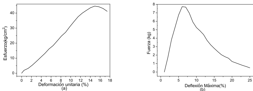
Figura 2: curvas para la combinación experimental de aglomerado N°7: (a) curva de esfuerzo deformación y (b) curva de flexión
