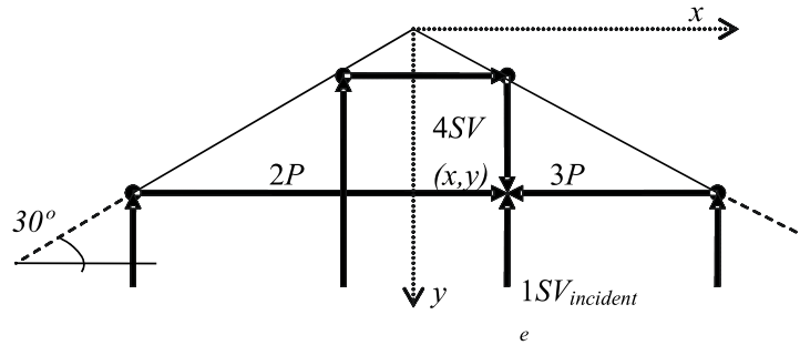
Fig. 7. Incidencia vertical de frente plano SV sobre una cuña infinita de 30°
