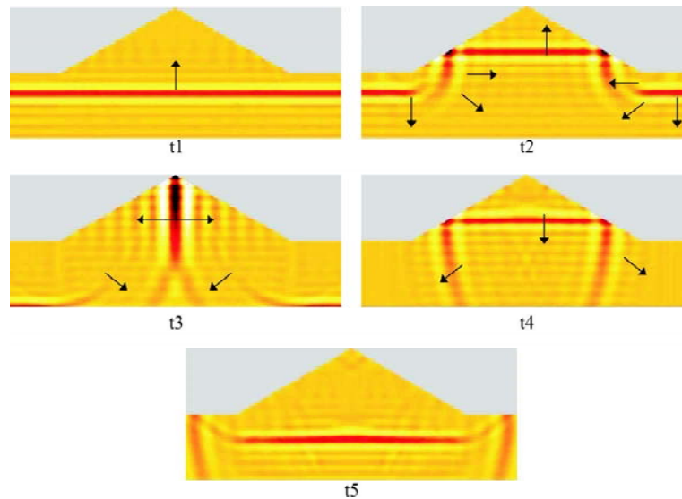
Fig. 10. Secuencia de propagación del movimiento horizontal debido a la incidencia vertical de un pulso de Ricker SV en una cuña finita de 30^\circ
