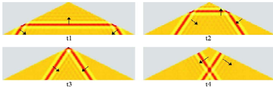
Fig. 4. Secuencia de la propagación vertical de un pulso de Ricker SH en una cuña infinita de 30^\circ
