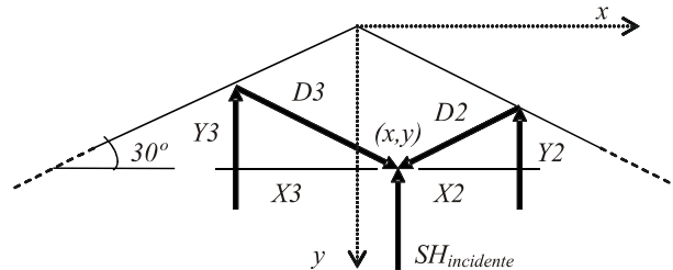
Fig. 2. Incidencia vertical de un frente plano SH sobre una cuña infinita de 30^\circ
