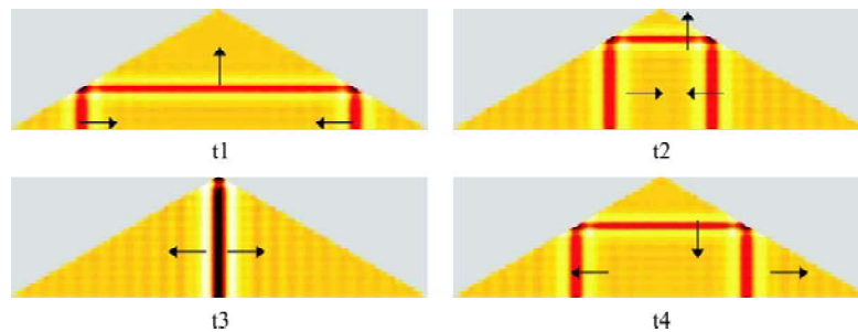
Fig. 8. Secuencia de propagación vertical de un pulso de Ricker SV en una cuña infinita de 30°
