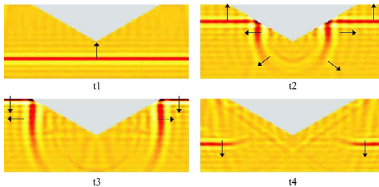
Fig. 13. Secuencia de propagación de la componente horizontal del movimiento debido a la incidencia vertical de un pulso de Ricker SV en un valle triangular
