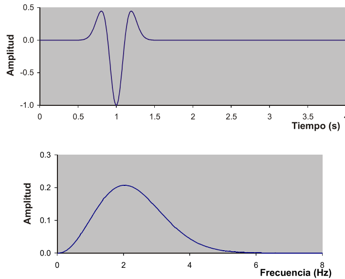
Fig. 3. Pulso de Ricker y su espectro de amplitudes de Fourier
