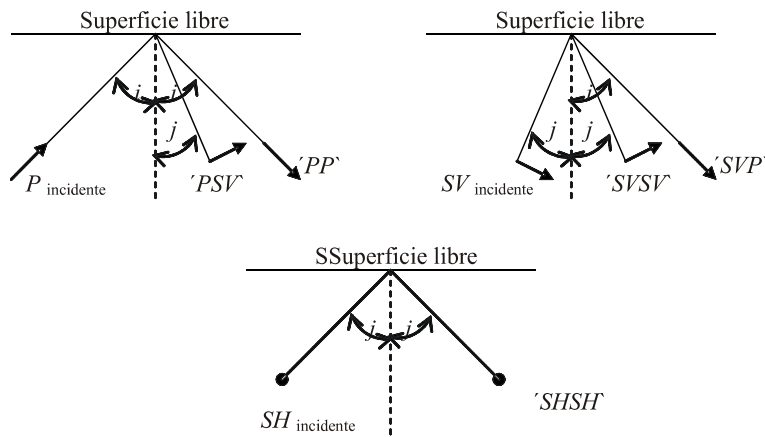
Fig. 1. Reflexión de ondas planas sobre una superficie libre
