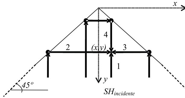
Fig. 5. Incidencia vertical de frente plano SH sobre una cuña infinita de 45^\circ
