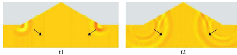
Fig. 11. Secuencia de propagación de la componente vertical del movimiento debido a la incidencia vertical de un pulso de Ricker SV en una cuña finita de 30^\circ
