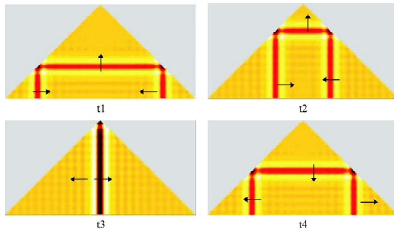
Fig. 6. Secuencia de propagación vertical de un pulso de Ricker SH en una cuña infinita de 45^\circ
